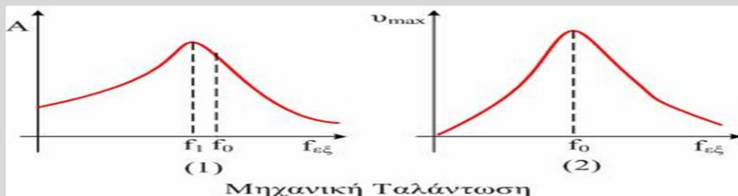
Μηχανική Ταλάντωση
