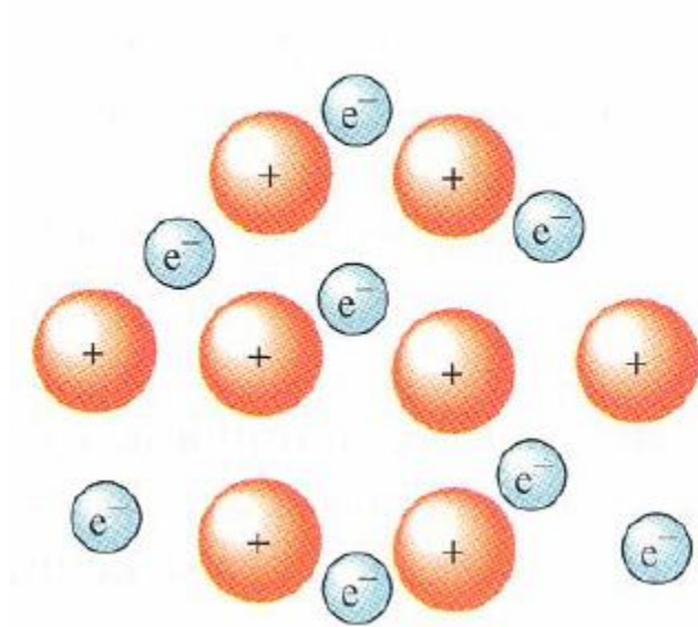
Αλκαλικό μέταλλο με ένα e - σθένους
