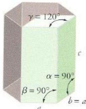
Εξαγωνικό
