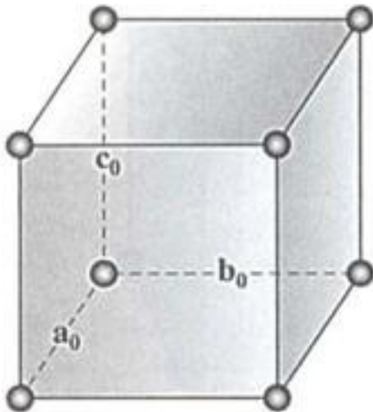
sc
