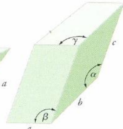
Τρικλινές
