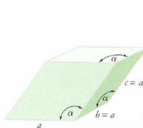
Ρομβοεδρικό
