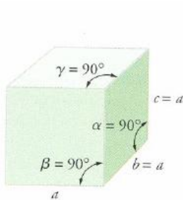
Κυβικό
