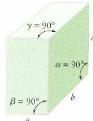
Ορθορομβικό
