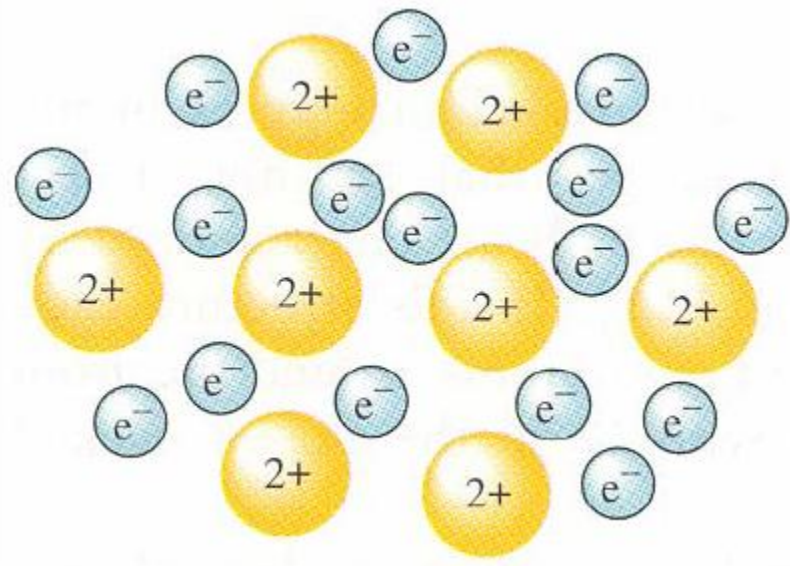
Αλκαλική γαία με δύο e - σθένους
