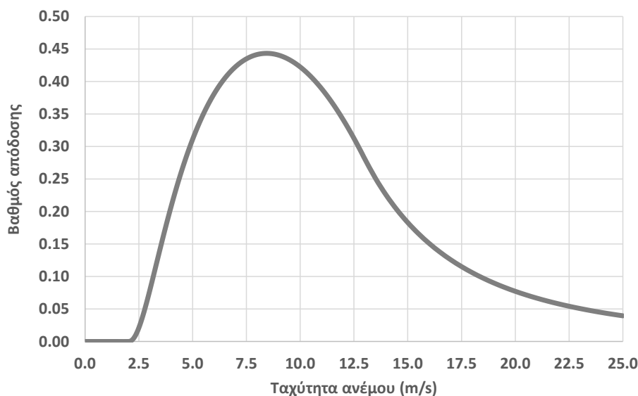
Εικόνα 2: Καμπύλη μεταβολής βαθμού απόδοσης συναρτήσει της ταχύτητας ανέμου.
