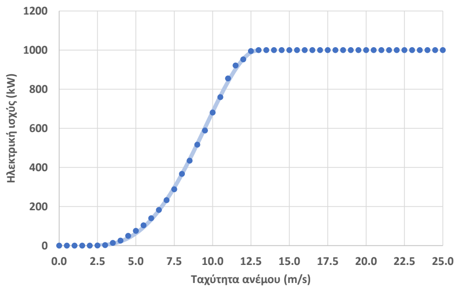
Εικόνα 1: Χαρακτηριστικά σημεία της καμπύλης ισχύος και προσαρμογή της αναλυτικής σχέσης (1) στο μη γραμμικό της τμήμα.
