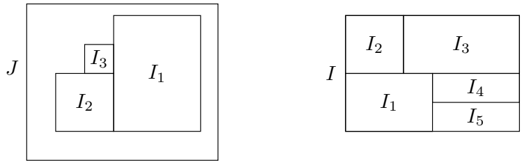
Σχήμα 3.1: Λήμμα 3.1.6 (ii)
