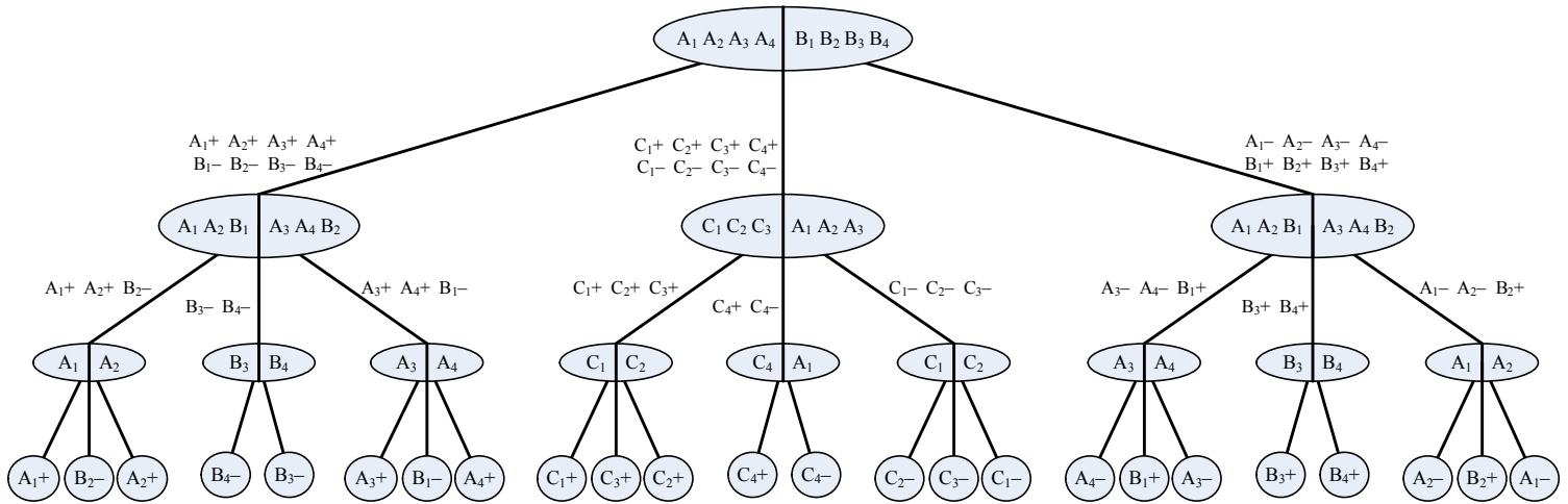
Σχήμα 1. Ένας “αλγόριθμος” που με 3 ζυγίσσεις βρίσκει το κάλπικο ανάμεσα σε 12 νομίσματα και αν αυτό είναι ελαφρύτερο ή βαρύτερο. Ο “αλγόριθμος” χωρίζει αρχικά τα νομίσματα σε 3 τετράδες: την τετράδα A με τα νομίσματα A_1, A_2, A_3, A_4 , την τετράδα B με τα νομίσματα B_1, B_2, B_3, B_4 , και την τετράδα C με τα νομίσματα C_1, C_2, C_3, C_4 . Η αναπαράσταση του αλγόριθμου βασίζεται σε ένα τριαδικό δέντρο συγκρίσεων. Κάθε κόμβος (εκτός από τα φύλλα) δηλώνει ότι τα νομίσματα στα αριστερά ζυγίζονται με τα νομίσματα στα δεξιά (π.χ. η ρίζα δηλώνει ότι τα νομίσματα της τετράδας A ζυγίζονται με αυτά της τετράδας B ). Αν η ζυγαριά γείρει αριστερά (αντ. δεξιά), ακολουθείται ο αριστερός (αντ. δεξιός) κλάδος, και αν η ζυγαριά ισορροπήσει, ακολουθείται ο μεσαίος κλάδος. Σε κάθε κλάδο σημειώνονται τα πιθανά ενδεχόμενα με βάση την διαθέσιμη πληροφορία από τις ζυγίσσεις. Η αναφορά σε ένα νόμισμα δηλώνει ότι αυτό μπορεί να είναι το κάλπικο, και το + (αντ. - ) δηλώνει ότι θα είναι βαρύτερο (αντ. ελαφρύτερο) από τα κανονικά (π.χ. τα ενδεχόμενα που αντιστοιχούν στον ψηλότερο αριστερό κλάδο είναι κάποιο από τα νομίσματα της τετράδας A να είναι κάλπικο και βαρύτερο από τα κανονικά ή κάποιο από τα νομίσματα της τετράδας B να είναι κάλπικο και ελαφρύτερο από τα κανονικά). Περιορίζοντας διαδοχικά τα ενδεχόμενα σε κάθε κλάδο, καταλήγουμε σε μοναδικό αποτέλεσμα σε κάθε φύλλο.
