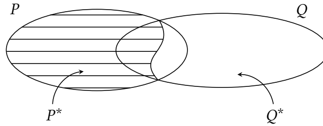
Διάγραμμα 3.5: Το ζεύγος (P^*, Q^*) ανάγει το ζεύγος (P, Q)
