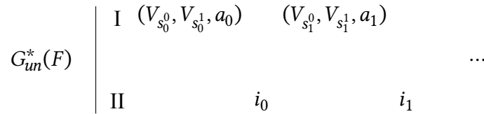
Διάγραμμα 7.6: Ο γύρος \sigma * \tau .
