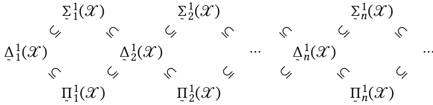
Διάγραμμα 3.2: Η ιεραρχία των προβολικών υποσυνόλων του \mathcal{X} .
