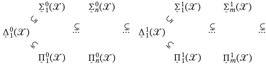
Διάγραμμα 3.3: Οι γνήσιοι εγκλεισμοί των ιεραρχιών των Borel (πεπερασμένης τάξης) και των προβολικών υποσυνόλων υπεραριθμήσιμου \mathcal{X} .
