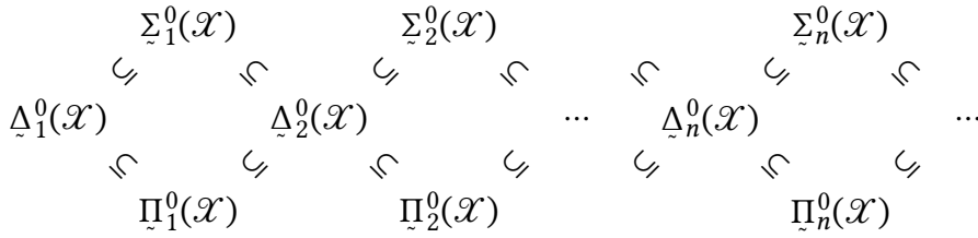
Διάγραμμα 3.1: Η ιεραρχία των Borel υποσυνόλων του \mathcal{X} πεπερασμένης τάξης.
