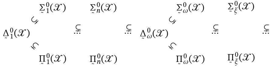
Διάγραμμα 4.3: Οι γνήσιοι εγκλεισμοί της ιεραρχίας των Borel συνόλων για υπεραριθμήσιμο \mathcal{X} .
