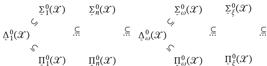
Διάγραμμα 4.1: Η ιεραρχία των Borel υποσυνόλων του \mathcal{X} .
