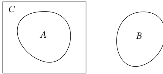
Διάγραμμα 3.6: Το C διαχωρίζει το A από το B
