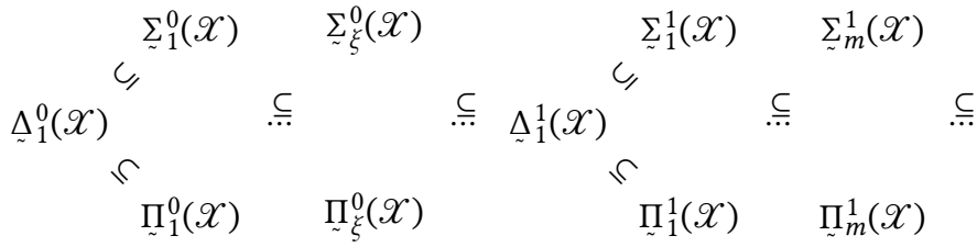
Διάγραμμα 4.2: Οι ιεραρχίες των Borel και των προβολικών υποσυνόλων του \mathcal{X} .
