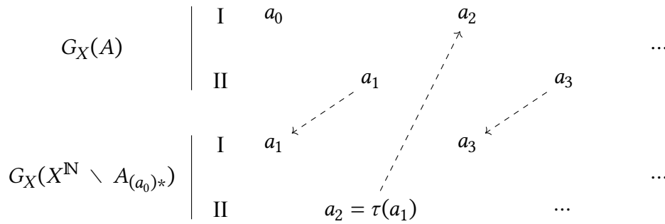
Διάγραμμα 7.4: Από το G_X(X^{\mathbb{N}} \setminus A_{(a_0)*}) στο G_X(A) .
