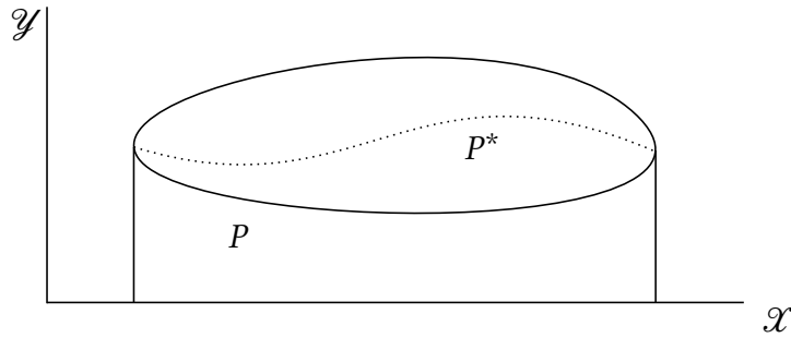
Διάγραμμα 3.4: Ενοποίηση του P από το P^*
