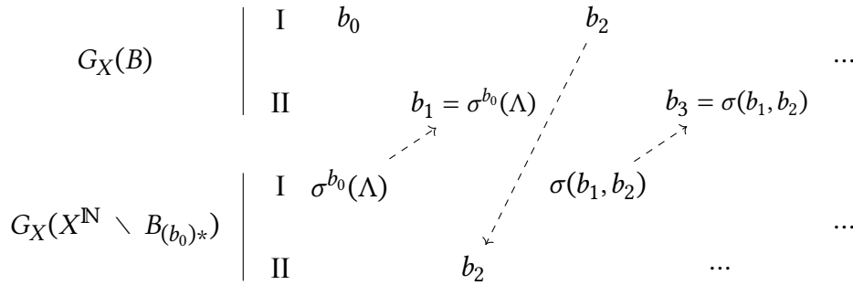
Διάγραμμα 7.5: Από το G_X(X^{\mathbb{N}} \setminus B_{(b_0)*}) στο G_X(B) .
