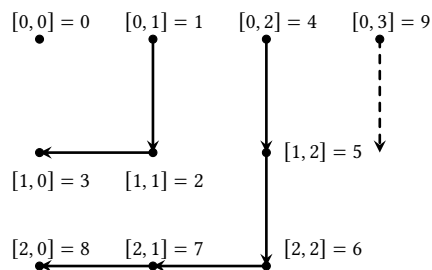
Διάγραμμα 5.1: Η “τετραγωνική” απαρίθμηση του \mathbb{N}^2
