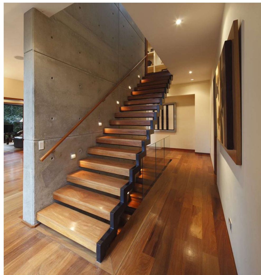
Σκάλα με ξύλινα σκαλοπάτια και μεταλλικό σκελετό, πακτωμένη σε τοίχιο από εμφανές σκυρόδεμα σε μονοκατοικία στο Περού. Φωτογραφία Juan Solano., , Περιοδικό Κτίριο
