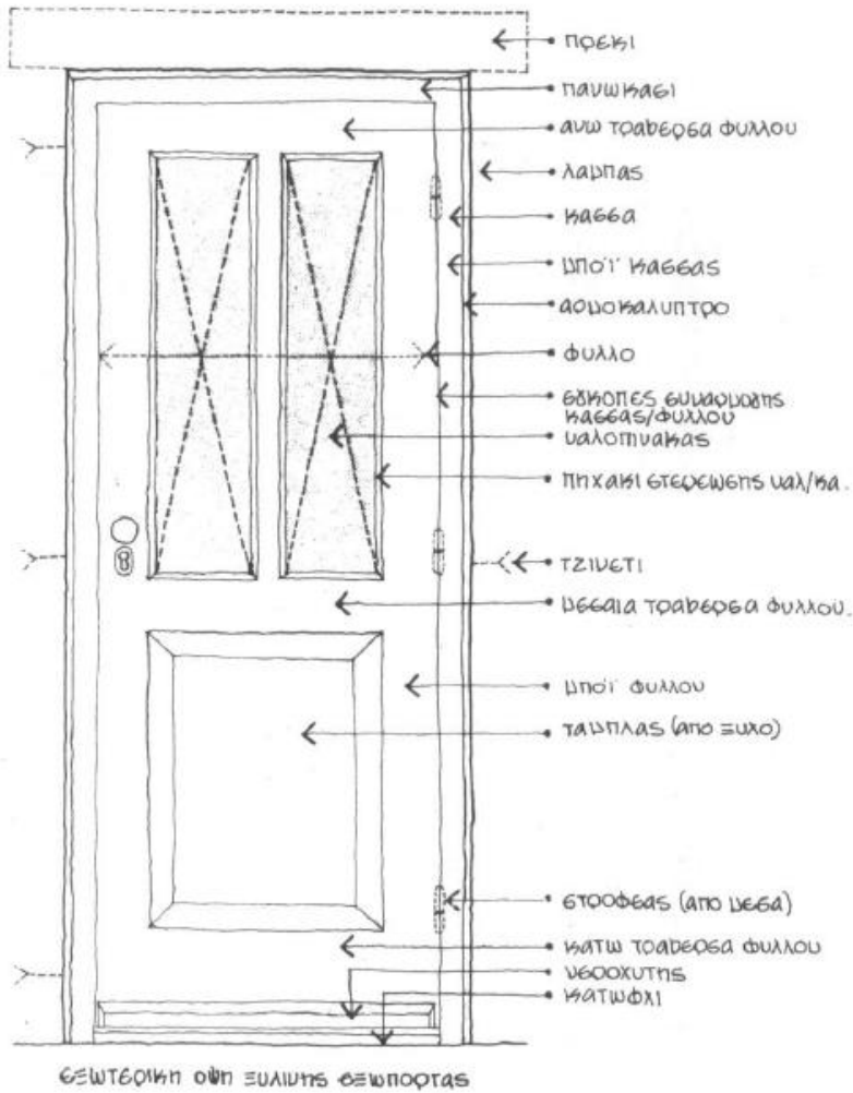
Σχ. 10.28. Τα κυριότερα κατασκευαστικά στοιχεία από τα οποία αποτελείται μια εξωτερική πόρτα και ένα παράθυρο.
