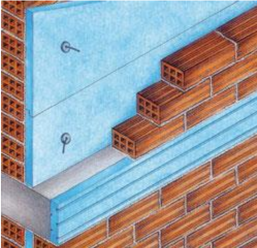
Οπτοπλινθοδομές
