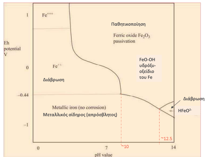
Απλοποιημένο διάγραμμα Pourbaix για τον Fe
