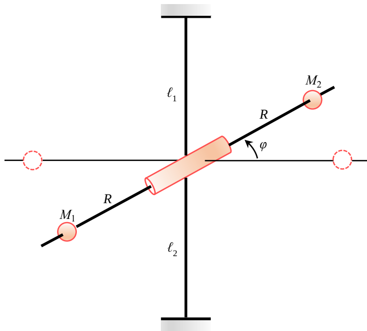
Σχήμα 4.5. Σχηματική παράσταση της πειραματικής διάταξης της άσκησης.
