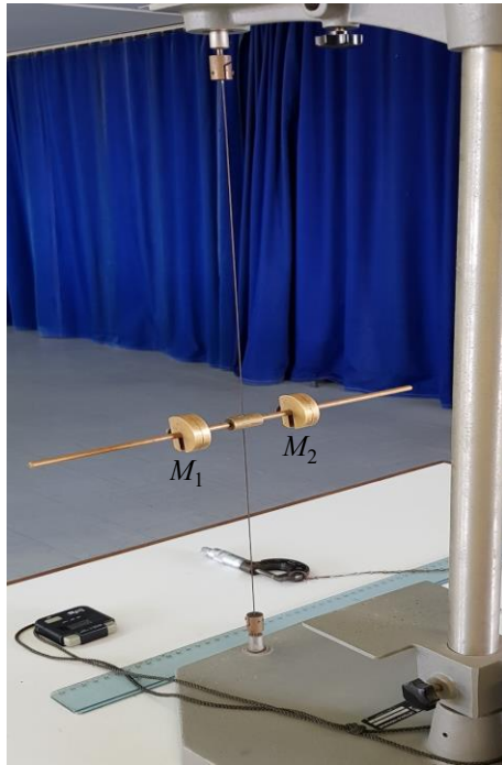
Σχήμα 4.6. Η διάταξη της άσκησης.
