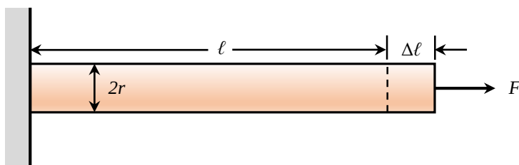
Σχήμα 4.1. Εφελκυσμός ράβδου. Η επιμήκυνση \Delta\ell σχεδιάστηκε υπερβολικά μεγάλη καθαρά για εποπτικούς λόγους. Κατά τη θλίψη, η δύναμη έχει αντίθετη φορά και συμπιέζει τη ράβδο κατά \Delta\ell .
