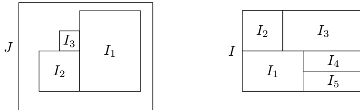
Σχήμα 3.1: Λήμμα 3.1.6 (ii)
