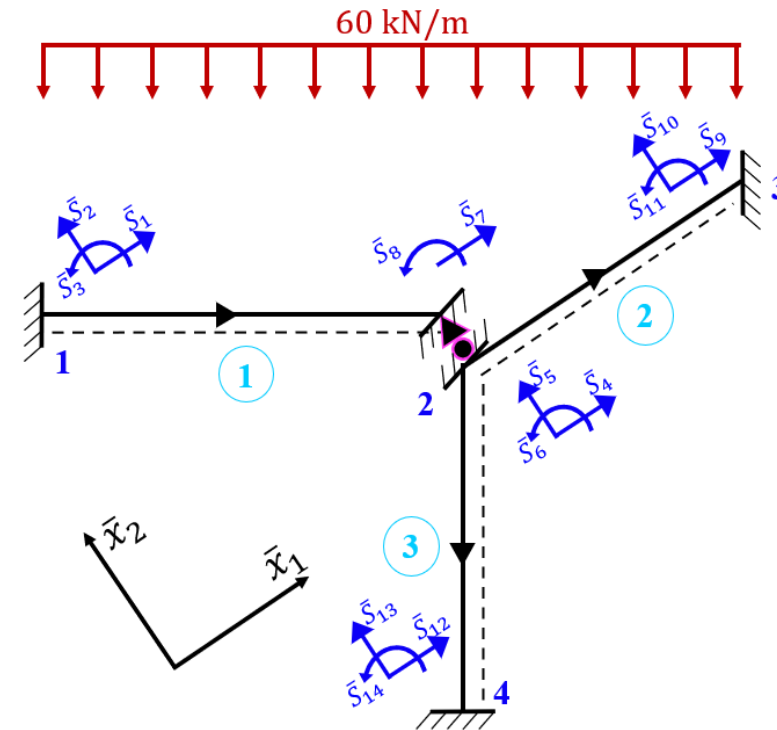
ΠΑΓΙΩΜΕΝΟΣ ΦΟΡΕΑΣ
