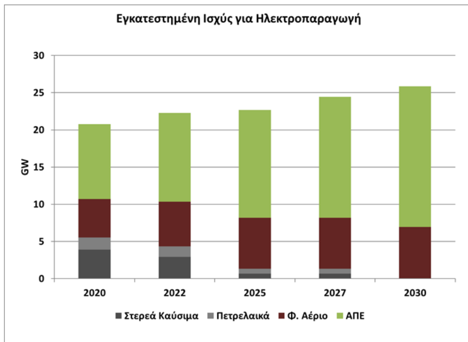
Διάγραμμα 31: Εξέλιξη της εγκατεστημένης ισχύος των μονάδων ηλεκτροπαραγωγής έως το έτος 2030.
