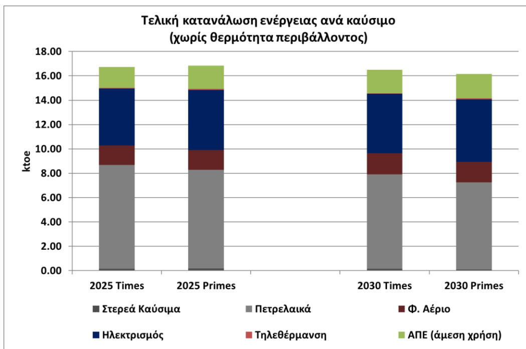
Διάγραμμα 56: Διαμόρφωση τελικής κατανάλωσης ενέργειας ανά καύσιμο έως το 2030 μεταξύ των διαφορετικών προσομοιώσεων (TIMES – PRIMES).
