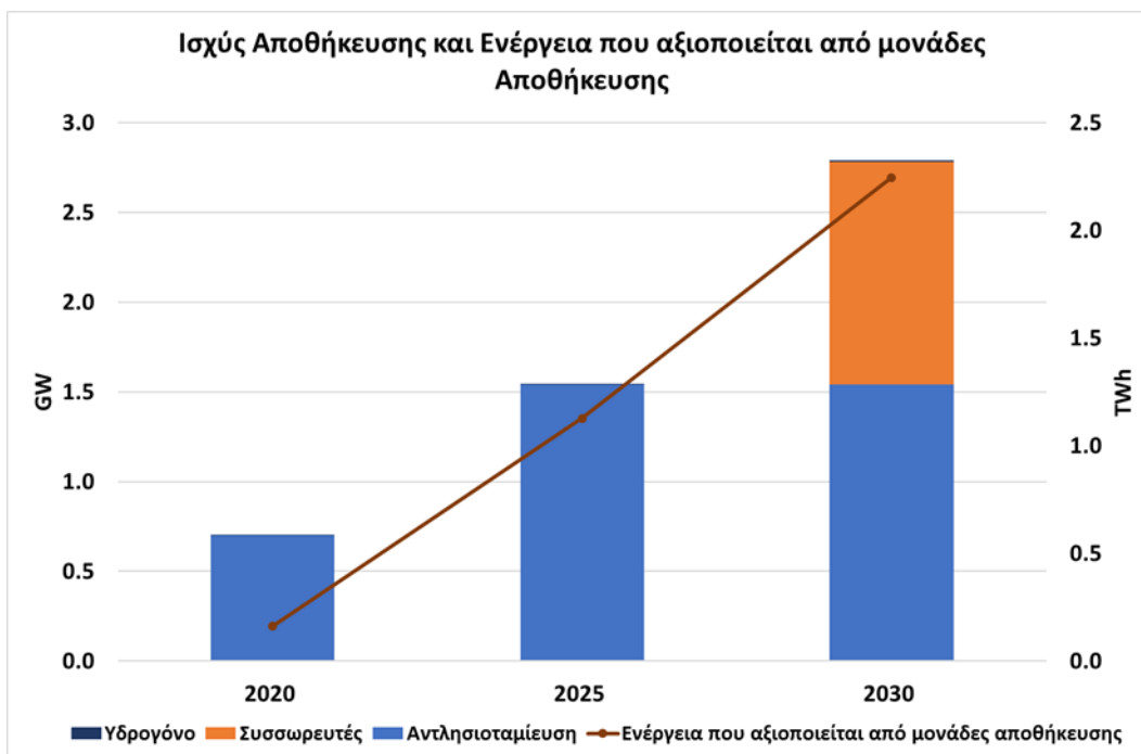
Διάγραμμα 33: Εξέλιξη της εγκατεστημένης ισχύος και ενέργειας για αποθήκευση έως το έτος 2030 σύμφωνα με το ενεργειακό μοντέλο PRIMES.
