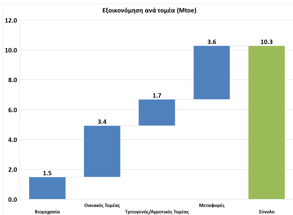
Διάγραμμα 39: Εξοικονόμηση ενέργειας ανά τομέα έως το έτος 2030 σε σύγκριση με την πρόβλεψη τελικής κατανάλωσης ανά τομέα του έτους 2007.
