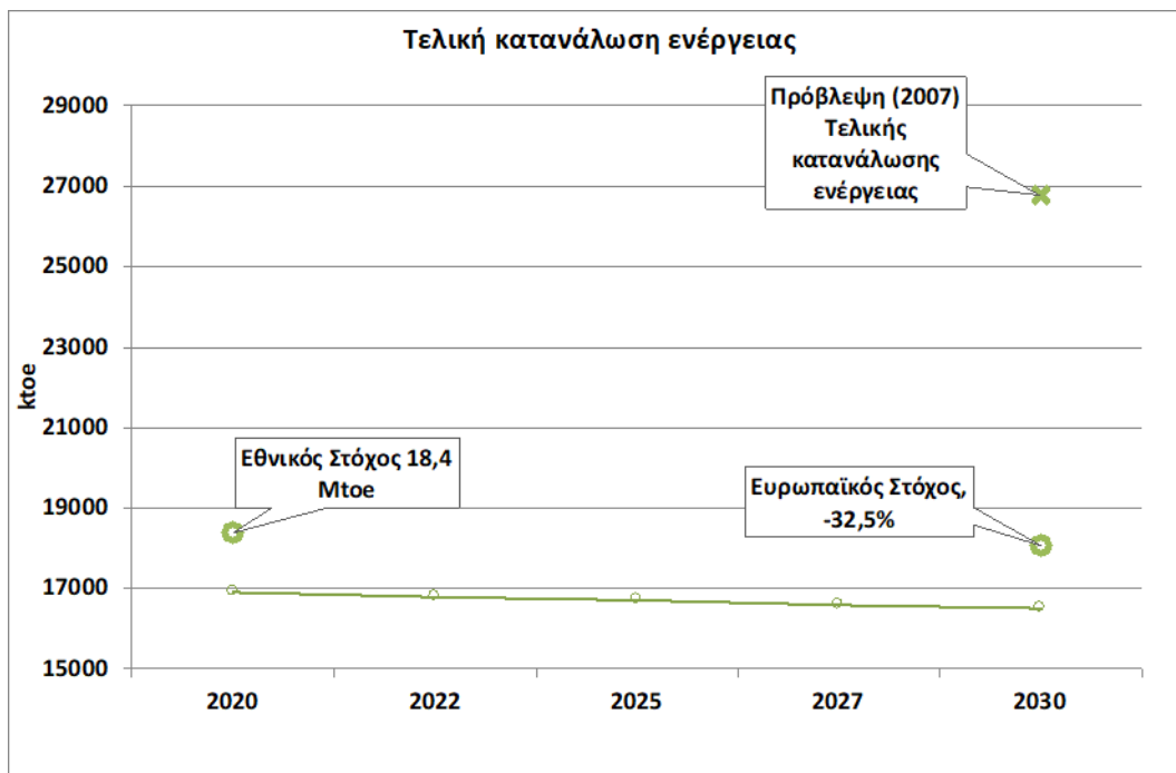
Διάγραμμα 27: Εξέλιξη τελικής κατανάλωσης ενέργειας έως το έτος 2030.
