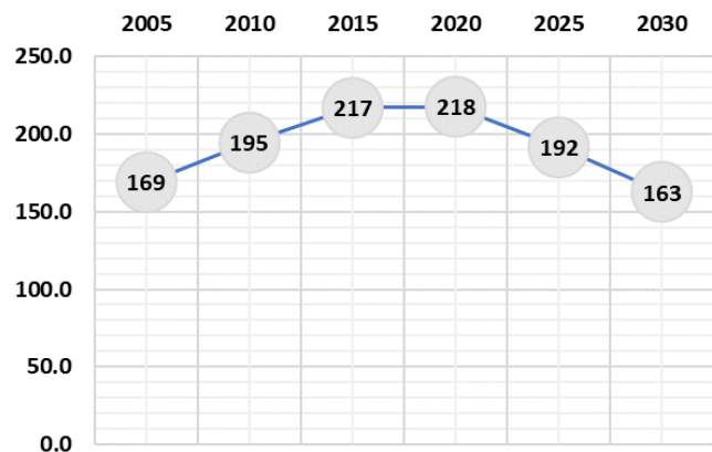
Ενεργειακή ένταση στη βιομηχανία (τιπ/εκ.€ προστ. Αξίας)
