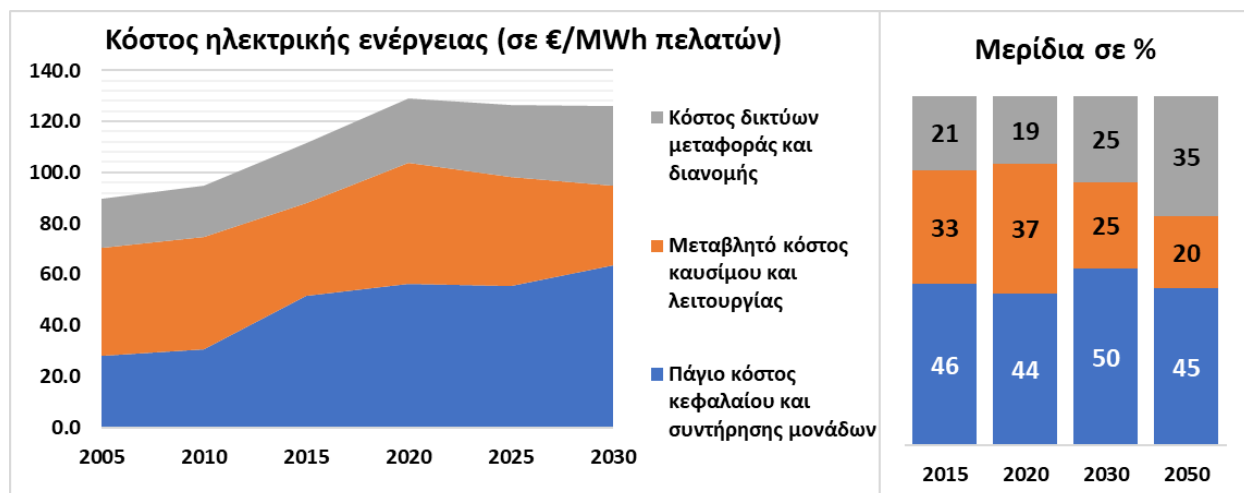
Διάγραμμα 59: Εξέλιξη κόστους ηλεκτρικής ενέργειας έως το έτος 2030.
