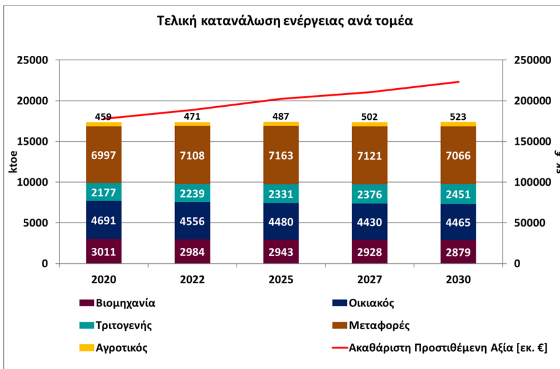
Διάγραμμα 37: Εξέλιξη τελικής κατανάλωσης ενέργειας ανά τομέα έως το έτος 2030.
