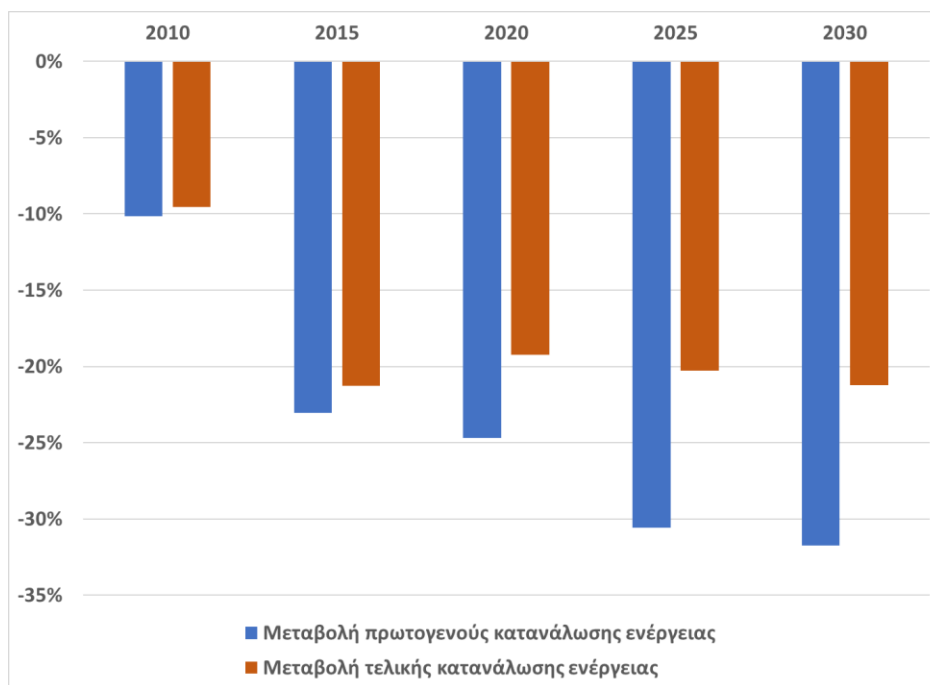
Διάγραμμα 40: Δείκτης βελτίωσης ενεργειακής απόδοσης σε σχέση με το έτος 2005.
