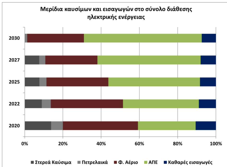
Διάγραμμα 34: Εξέλιξη της καθαρής παραγωγής και των εισαγωγών ηλεκτρικής ενέργειας έως το έτος 2030.
