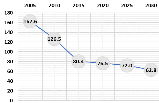
Μέση κατανάλωση ενέργειας στις οικίες (kWh/τμ)
