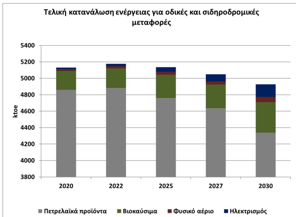
Διάγραμμα 44: Εξέλιξη τελικής κατανάλωσης ενέργειας στις οδικές και σιδηροδρομικές μεταφορές έως το έτος 2030.
