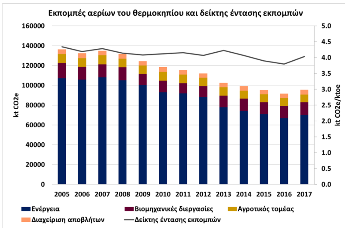
Διάγραμμα 8: Εξέλιξη εκπομπών αερίων του θερμοκηπίου ανά τομέα συνεισφοράς και δείκτη έντασης εκπομπών.
