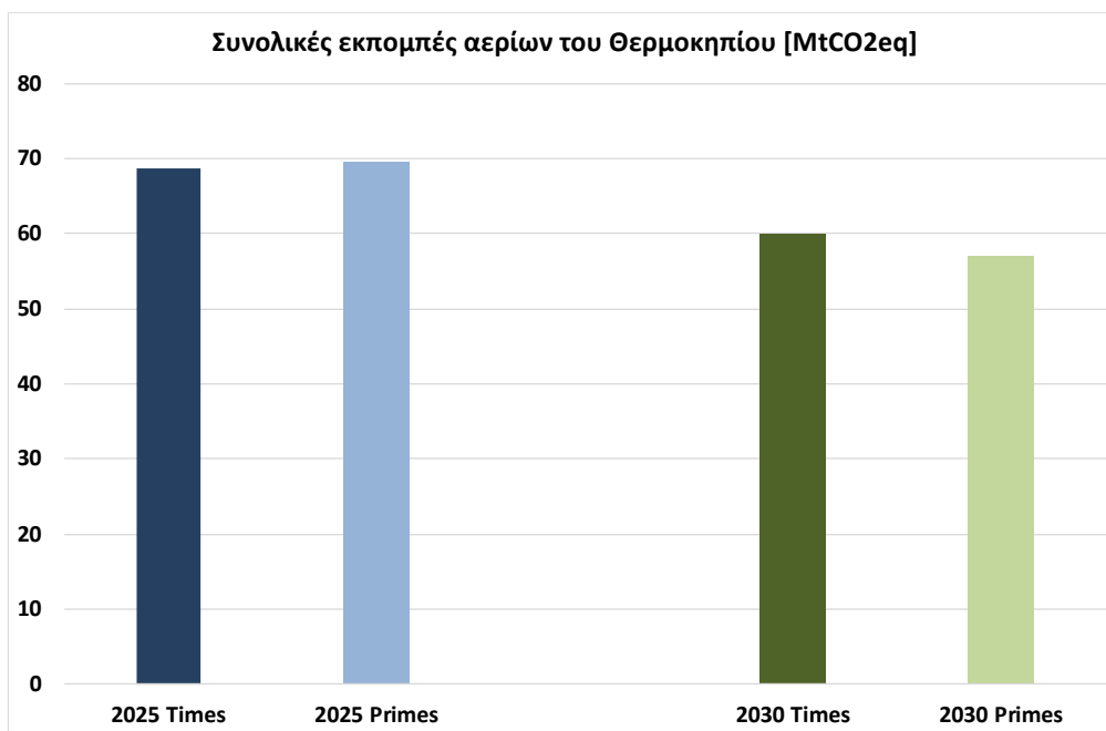
Διάγραμμα 48: Συνολικές εκπομπές αερίων θερμοκηπίου μεταξύ των διαφορετικών ενεργειακών προσομοιώσεων (TIMES – PRIMES).
