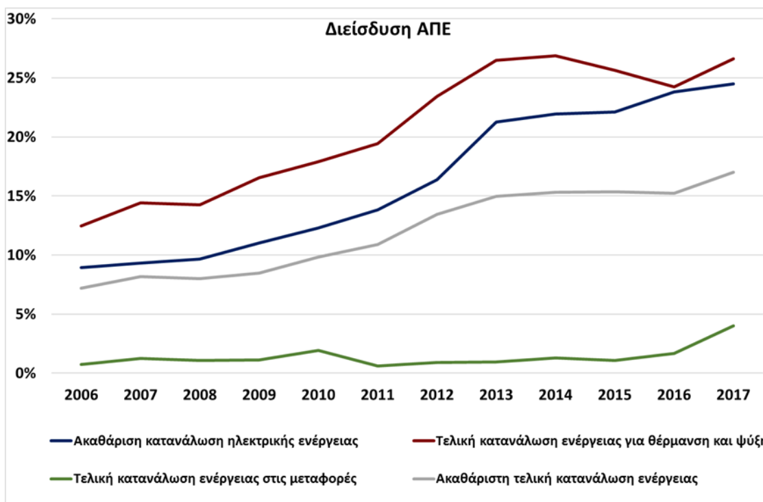
Διάγραμμα 12: Συνολικά και ειδικά μερίδια συμμετοχής των ΑΠΕ στο εγχώριο ενεργειακό σύστημα στη βάση μεθοδολογίας της Ευρωπαϊκής Ένωσης.
