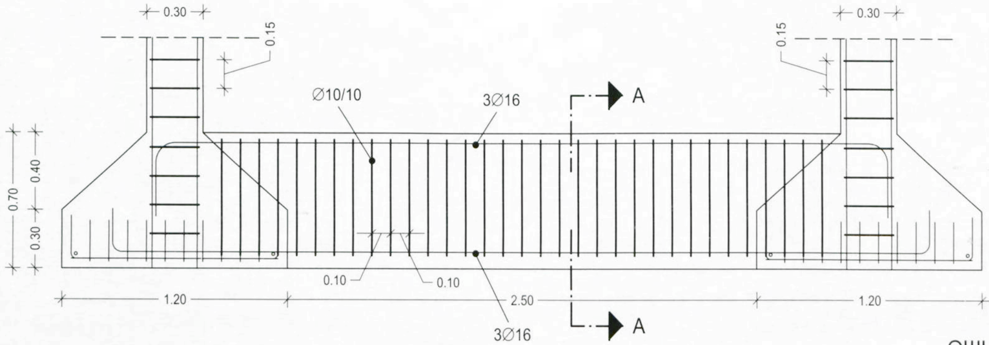
ΟΨΗ ΚΛ. 1:20
