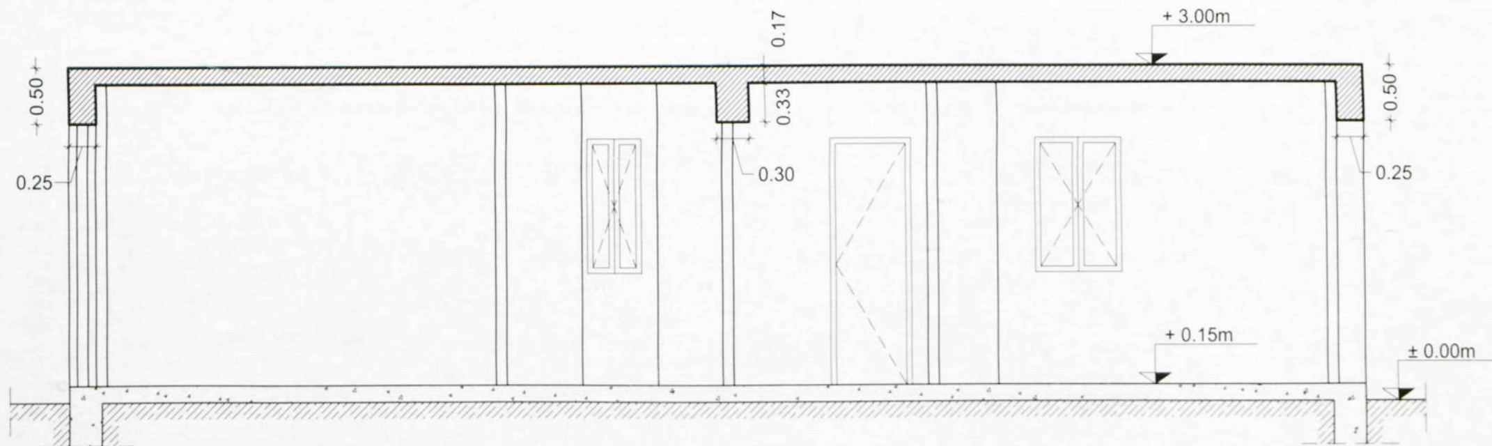
ΤΟΜΗ ΙΣΟΓΕΙΟΥ Α - Α ΚΛΙΜΑΚΑ 1:50
