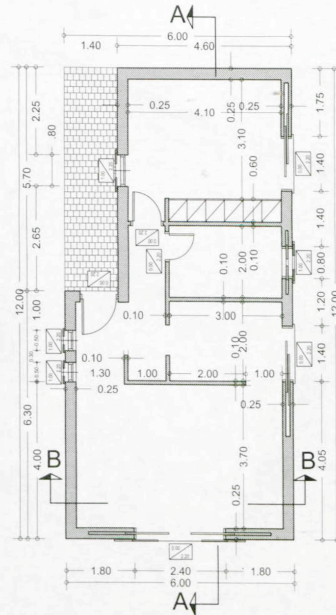
ΚΑΤΟΨΗ ΙΣΟΓΕΙΟΥ
