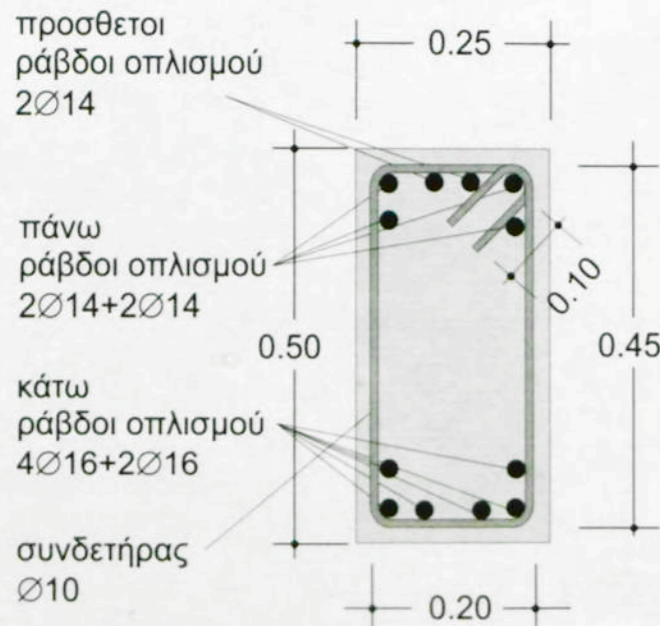
ΤΟΜΗ Α κλίμακα 1:10
