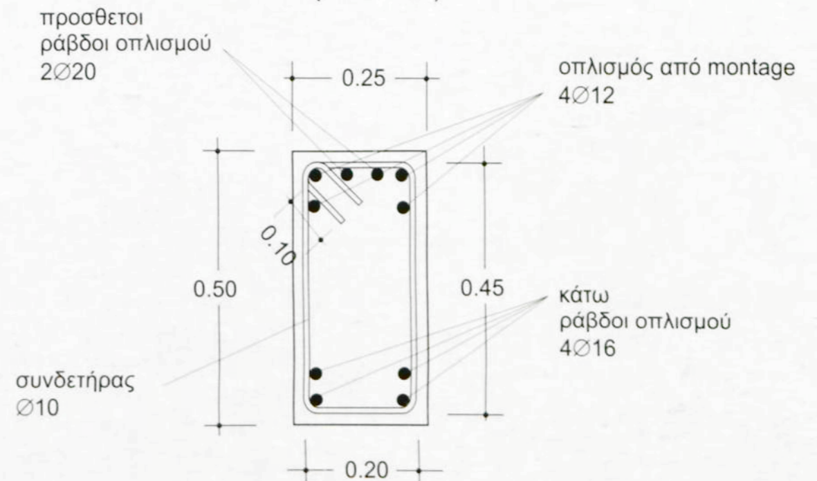
ΤΟΜΗ Β (Μεσαίας Στήριξης) κλίμακα 1:10)
