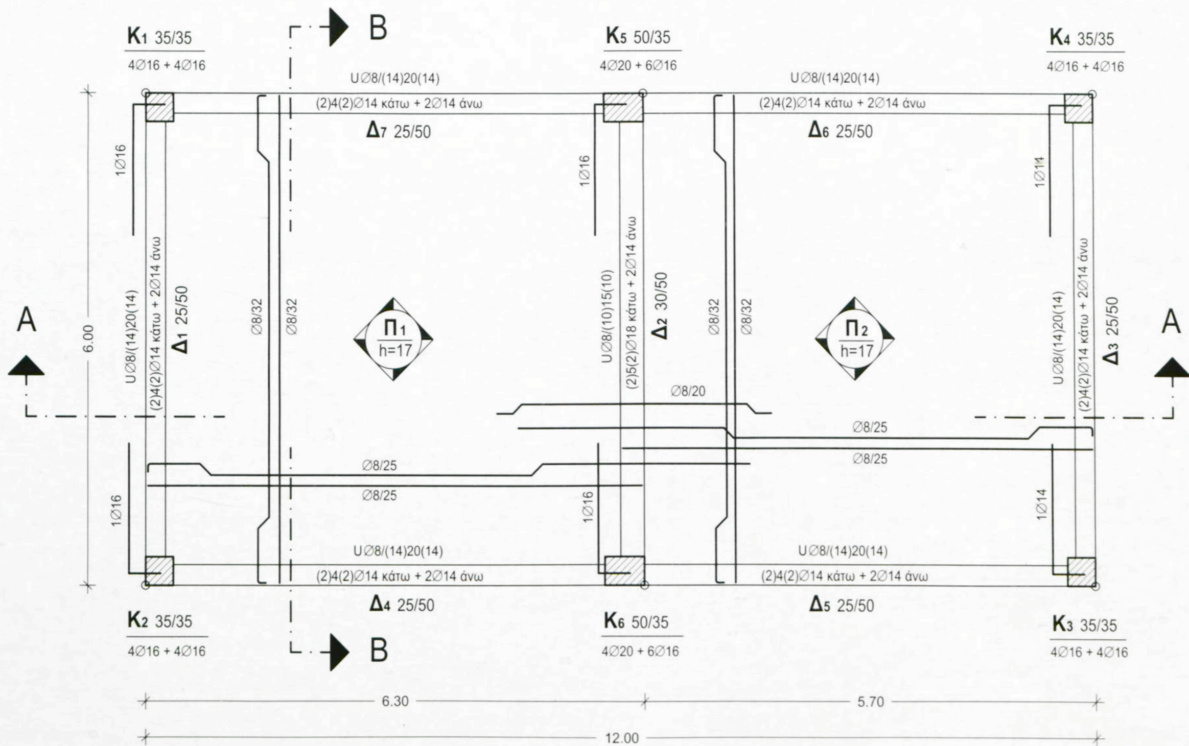
ΕΥΛΟΤΥΠΟΣ ΙΣΟΓΕΙΟΥ ΚΛΙΜΑΚΑ 1:50
