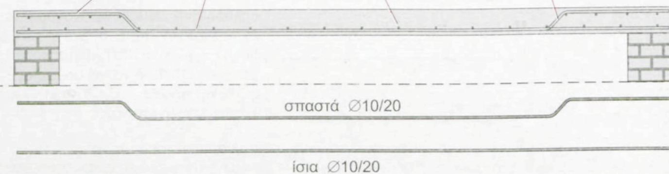
ΟΨΗ ΚΛΙΜΑΚΑ 1:25
