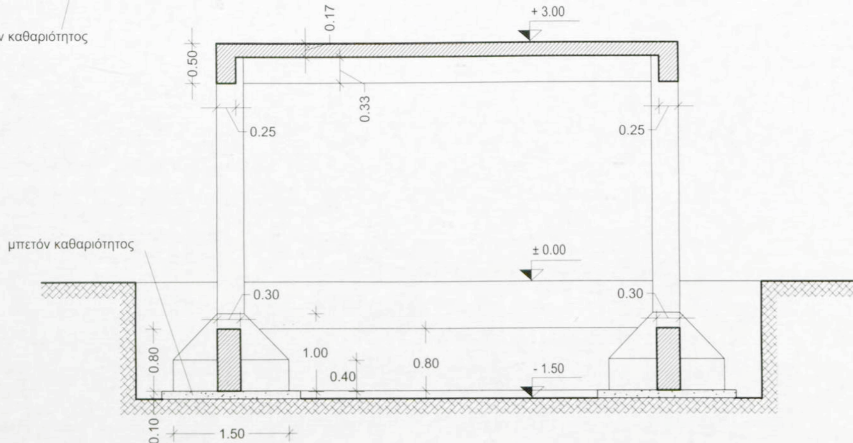
ΤΟΜΗ Α - Α ΚΛΙΜΑΚΑ 1:50
