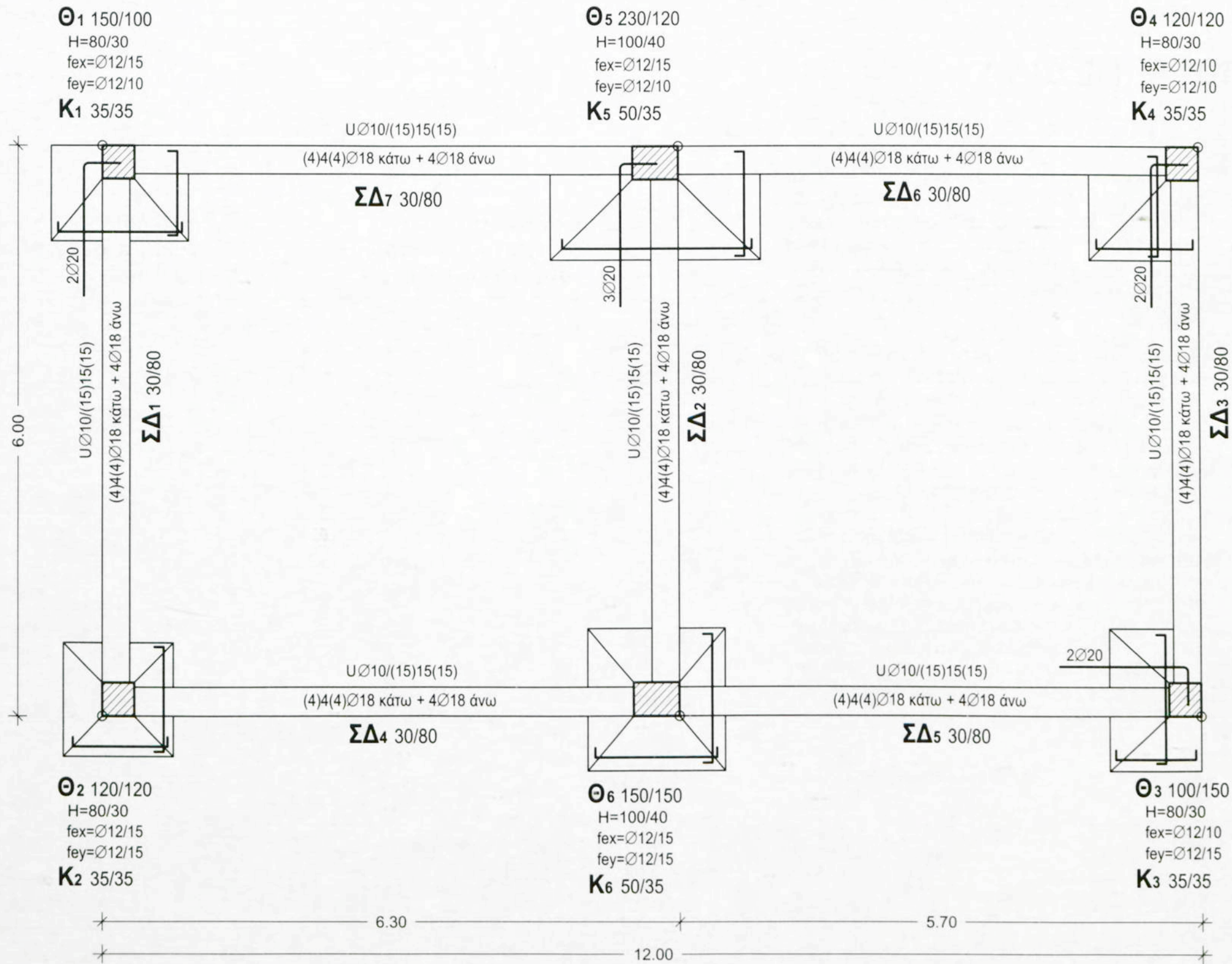
ΕΥΛΟΤΥΠΟΣ ΘΕΜΕΛΙΩΣΗΣ ΚΛΙΜΑΚΑ 1:50
