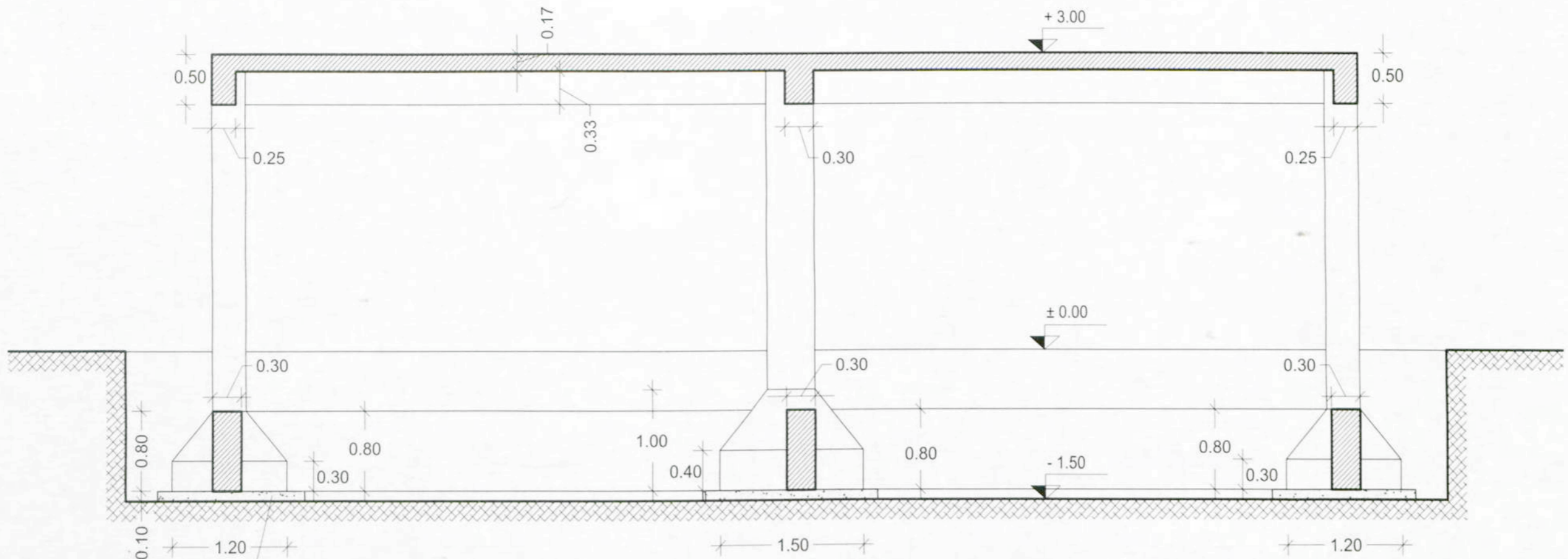
ΤΟΜΗ Α - Α ΚΛΙΜΑΚΑ 1:50
