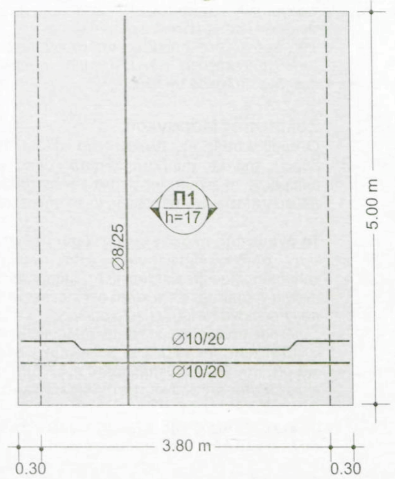
ΚΑΤΟΨΗ ΚΛΙΜΑΚΑ 1:50
