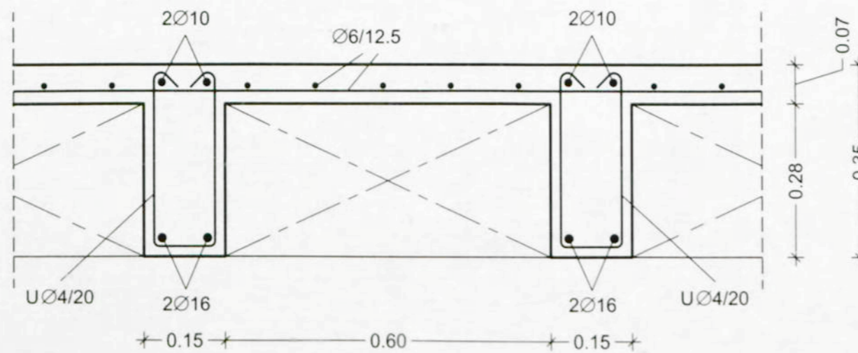
ΛΕΠΤΟΜΕΡΕΙΑ Α ΚΛ. 1:10
