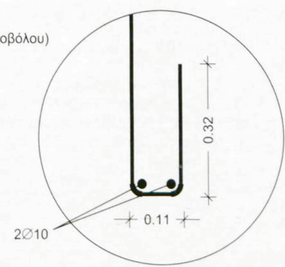
Λεπτομέρεια Α'
