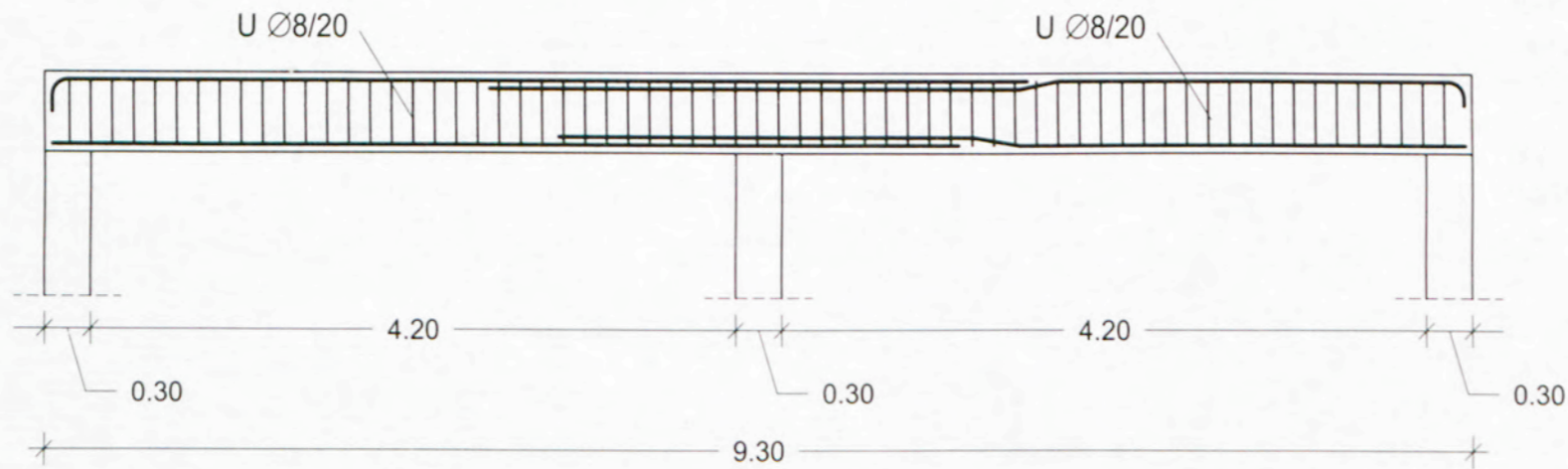
ΤΟΜΗ Κλίμακα 1:50
