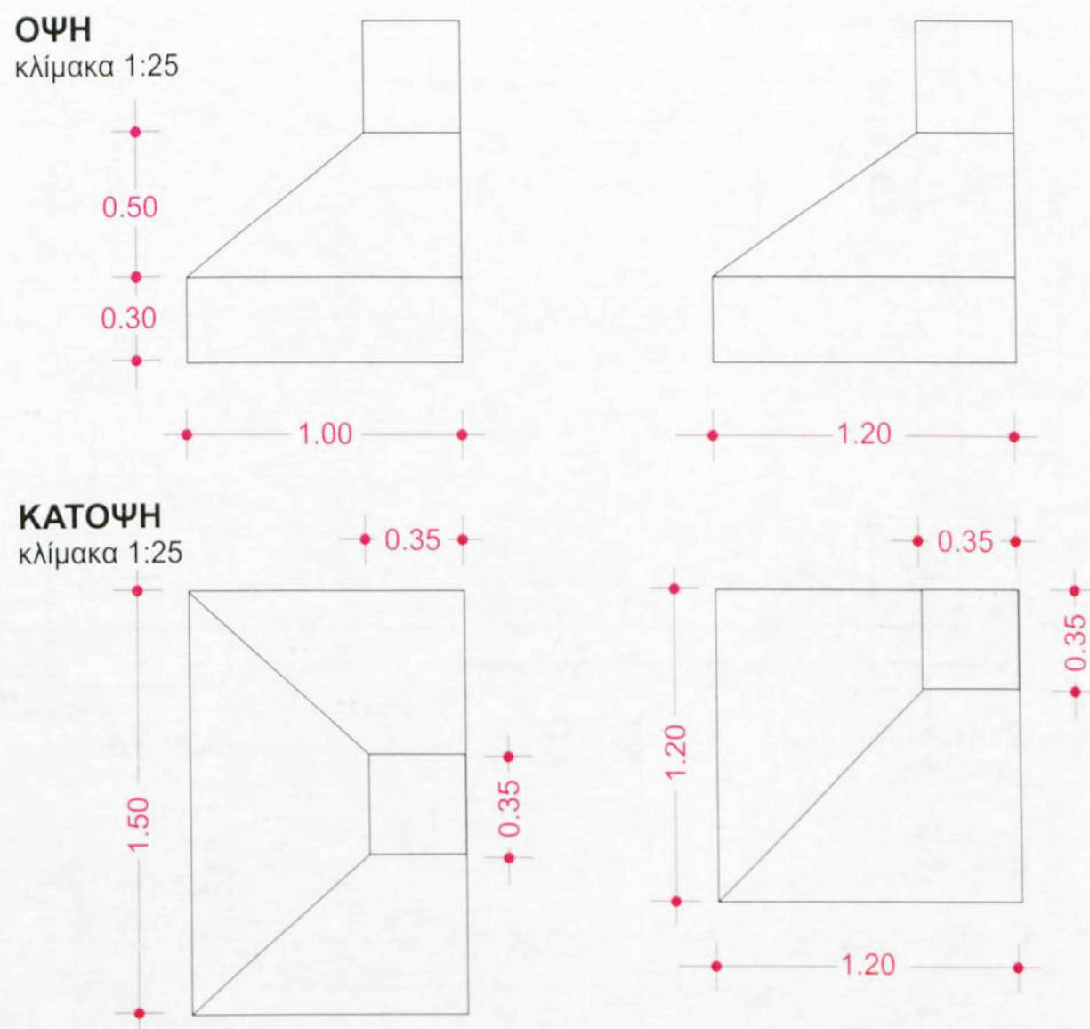
πέδιλο έκκεντρο κατά μία κατεύθυνση
