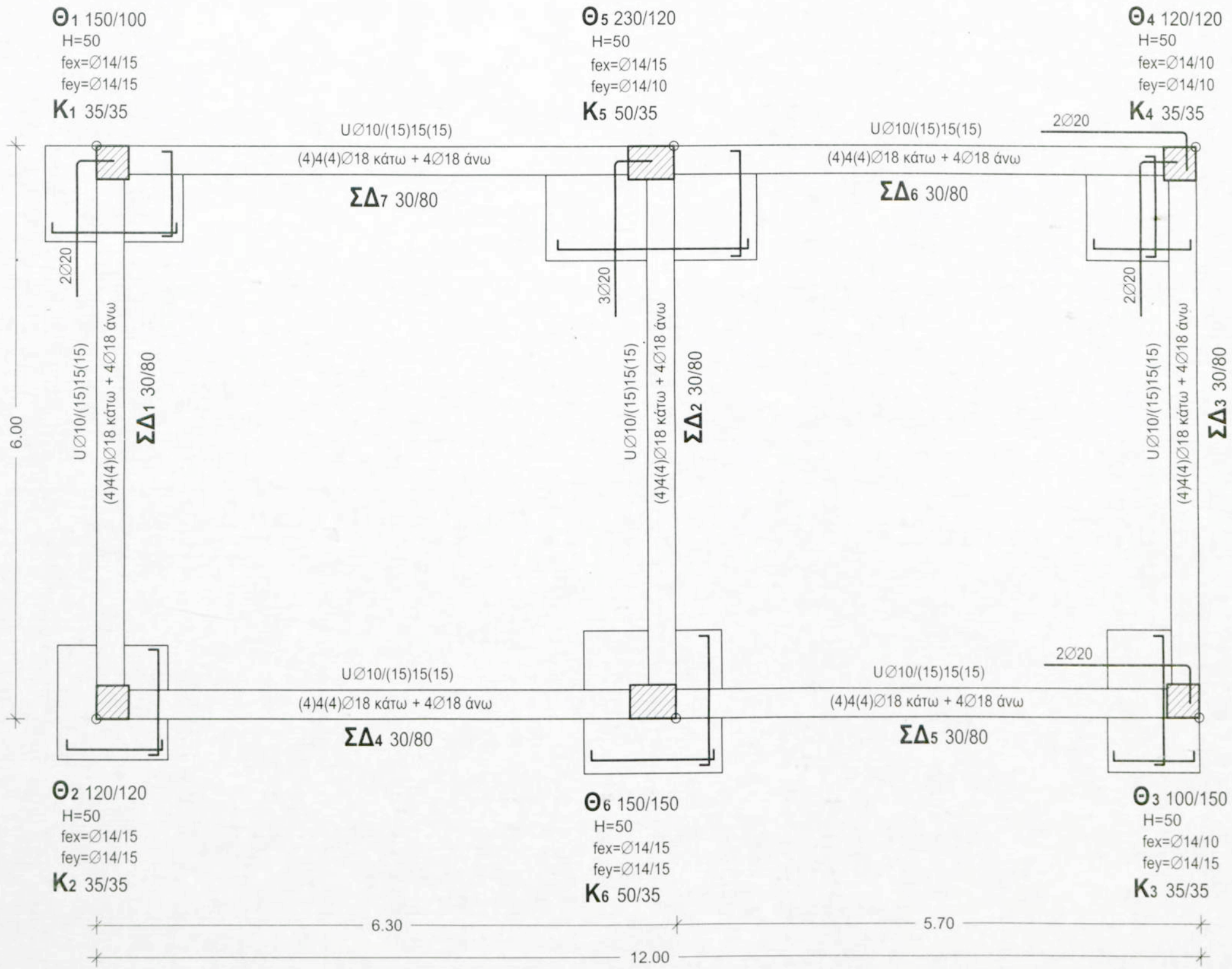
ΕΥΛΟΤΥΠΟΣ ΘΕΜΕΛΙΩΣΗΣ ΚΛΙΜΑΚΑ 1:50
