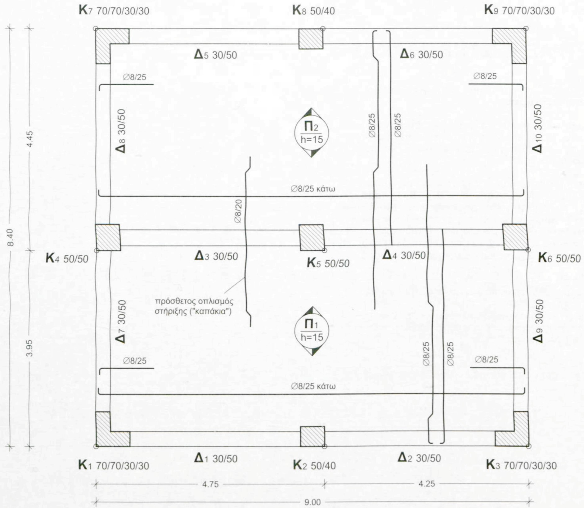
ΕΥΛΟΤΥΠΟΣ ΣΥΝΕΧΩΝ ΑΜΦΙΕΡΕΙΣΤΩΝ ΠΛΑΚΩΝ ΚΛΙΜΑΚΑ 1:50
