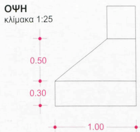
πέδιλο έκκεντρο κατά μία κατεύθυνση
