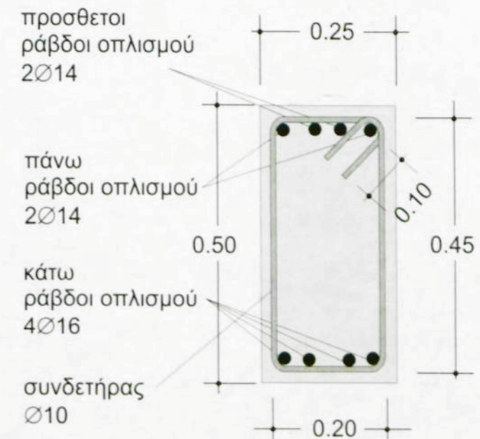
ΤΟΜΗ Γ κλίμακα 1:10
