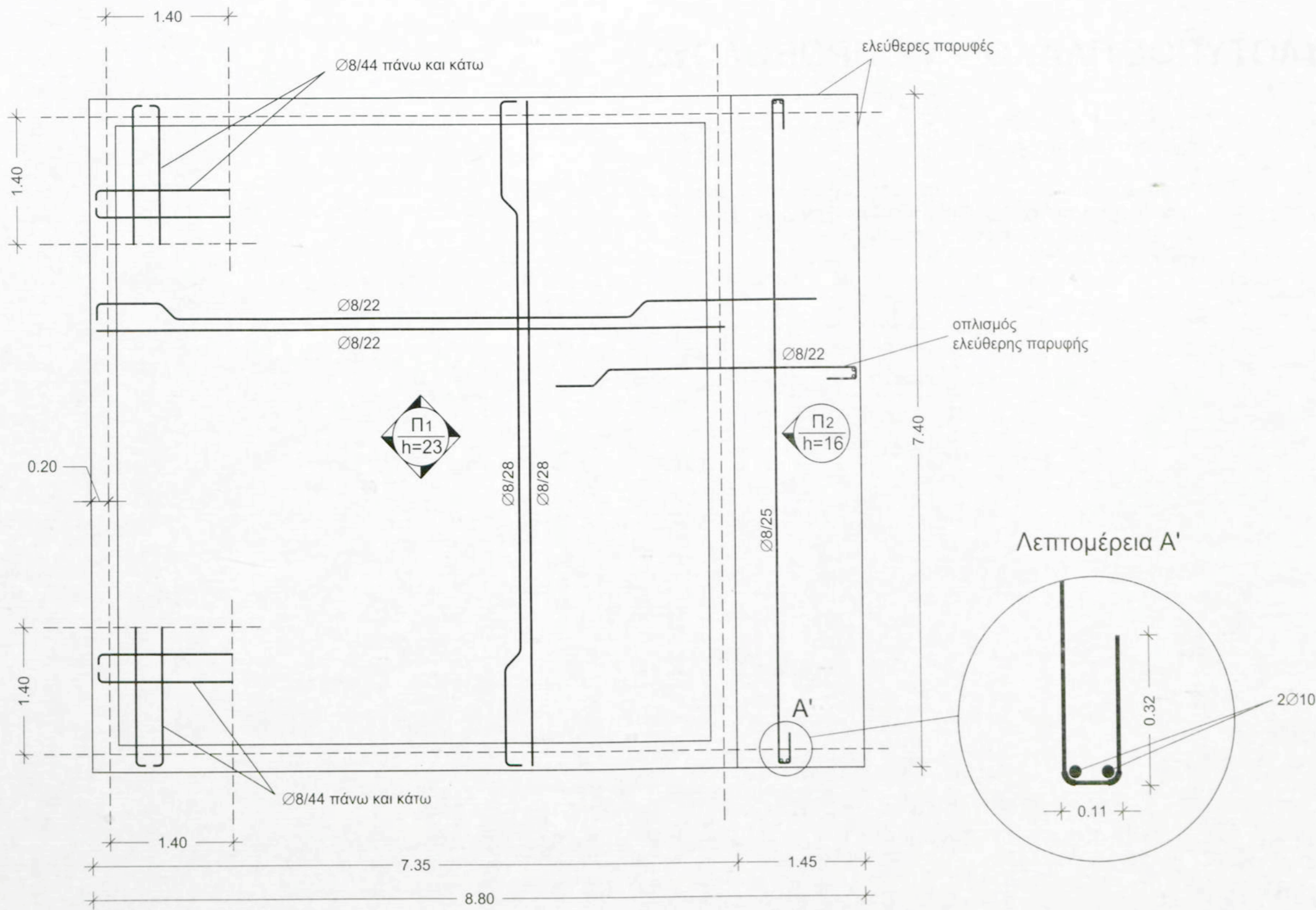
ΕΥΛΟΤΥΠΟΣ ΤΕΤΡΑΕΡΕΙΣΤΗΣ ΠΛΑΚΑΣ ΜΕ ΠΡΟΒΟΛΟ ΚΛΙΜΑΚΑ 1:50
