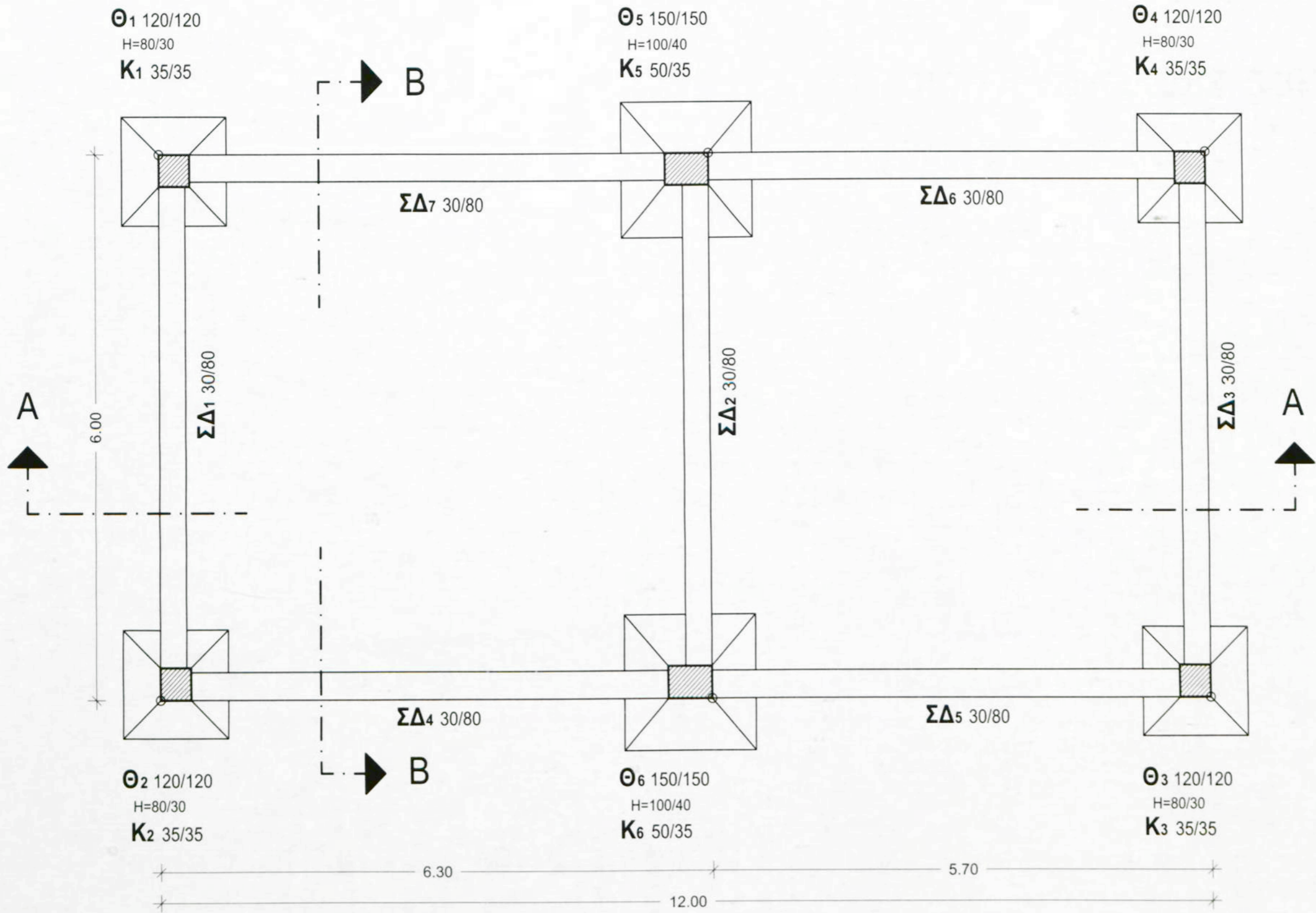
ΕΥΛΟΤΥΠΟΣ ΘΕΜΕΛΙΩΣΗΣ (ΜΑΡΑΓΚΟΥ) ΚΛΙΜΑΚΑ 1:50
