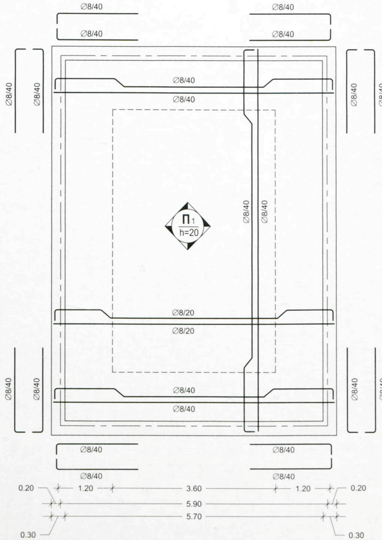
ΕΥΛΟΤΥΠΟΣ ΤΕΤΡΑΕΡΕΙΣΤΗΣ ΠΛΑΚΑΣ ΚΛΙΜΑΚΑ 1:50
