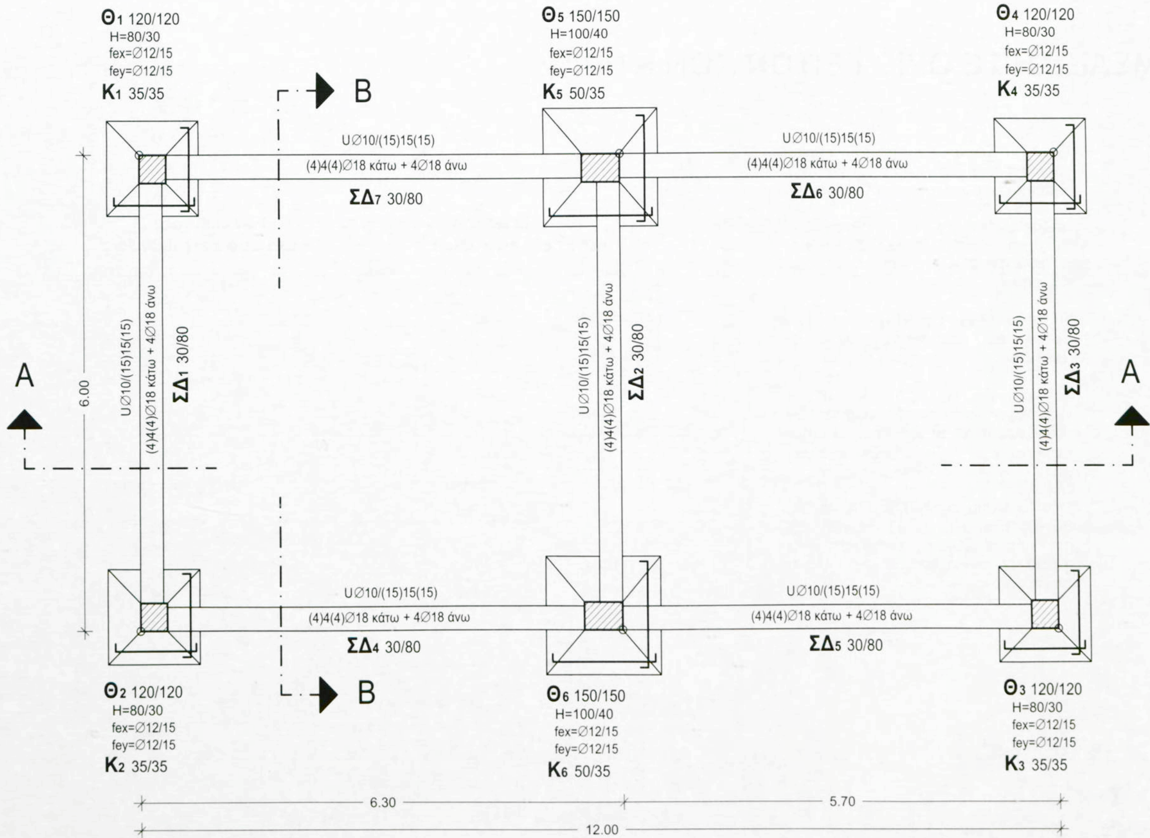
ΕΥΛΟΤΥΠΟΣ ΘΕΜΕΛΙΩΣΗΣ ΚΛΙΜΑΚΑ 1:50
