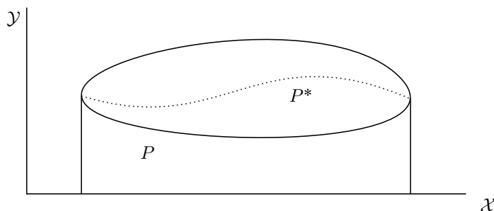
Διάγραμμα 4. Ομοιομορφοποίηση του P από το P^*
