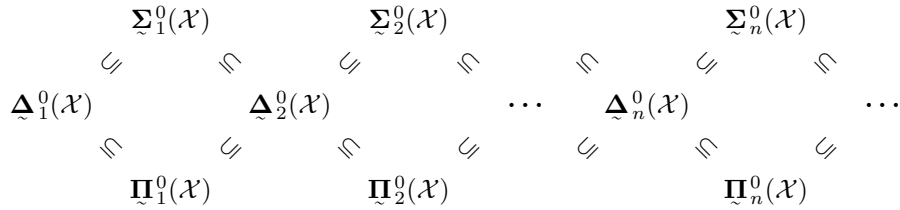
Διάγραμμα 1. Η ιεραρχία των Borel υποσυνόλων του \mathcal{X} πεπερασμένης τάξης.
