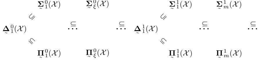
Διάγραμμα 8. Οι ιεραρχίες των Borel και των προβολικών υποσυνόλων του \mathcal{X} .
