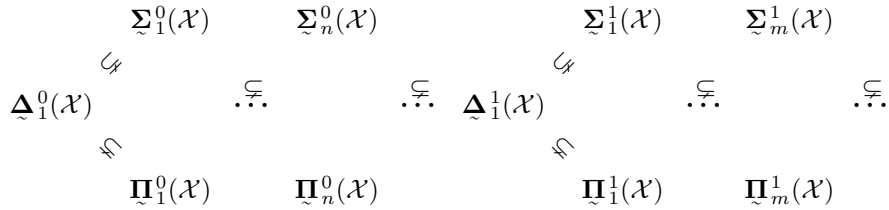
Διάγραμμα 3. Οι γνήσιοι εγκλεισμοί των ιεραρχιών των Borel (πεπερασμένης τάξης) και των προβολικών υποσυνόλων υπεραριθμήσιμου \mathcal{X} .
