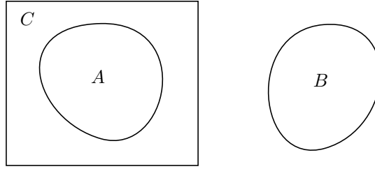
Διάγραμμα 6. Το C διαχωρίζει το A από το B
