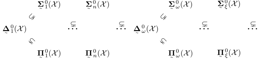
Διάγραμμα 9. Οι γνήσιοι εγκλεισμοί της ιεραρχίας των Borel συνόλων για υπεραριθμήσιμο \mathcal{X} .
