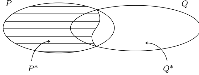
Διάγραμμα 5. Το ζεύγος (P^*, Q^*) ανάγει το ζεύγος (P, Q)
