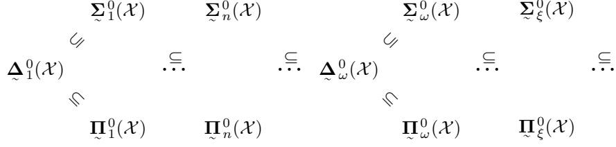
Διάγραμμα 7. Η ιεραρχία των Borel υποσυνόλων του \mathcal{X} .
