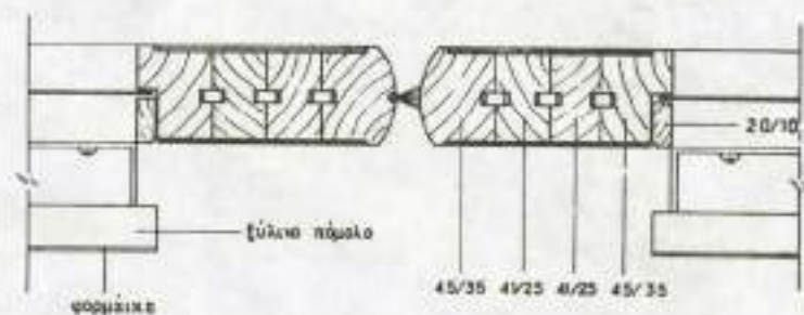
TOMH γ-γ
