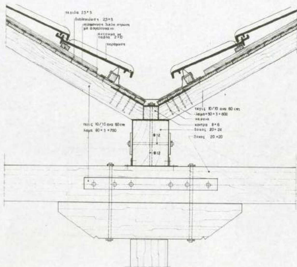
5.41.3. Λεπτομέρεια A13: αυλάκι
