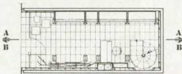
6.13.1. Κατόψεις και αξονομετρικές τομές του εσωτερικού χώρου
