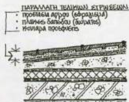
5.19.2. Συμβατική μόνωση σε βατό δώμα
