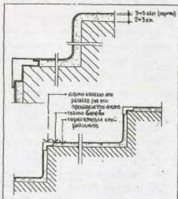
5.11.1. Επίστρωση πατημάτων με συνθετικά υλικά
