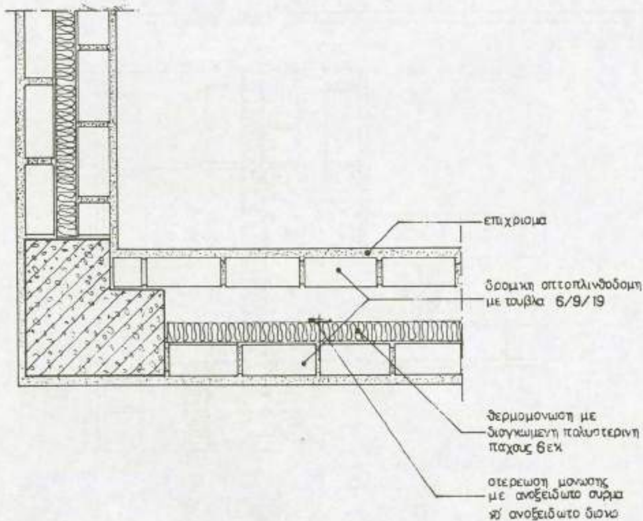
7.37. Λεπτομέρειες στρογγυλοδομών ( τούβλα ) σε κάτοψη
