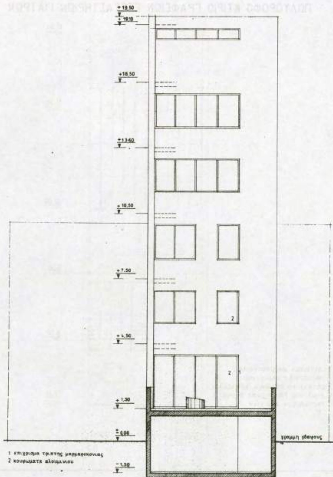
7.22. Όψη μεσημβρινή ( όψη στον σκάλυττο)
