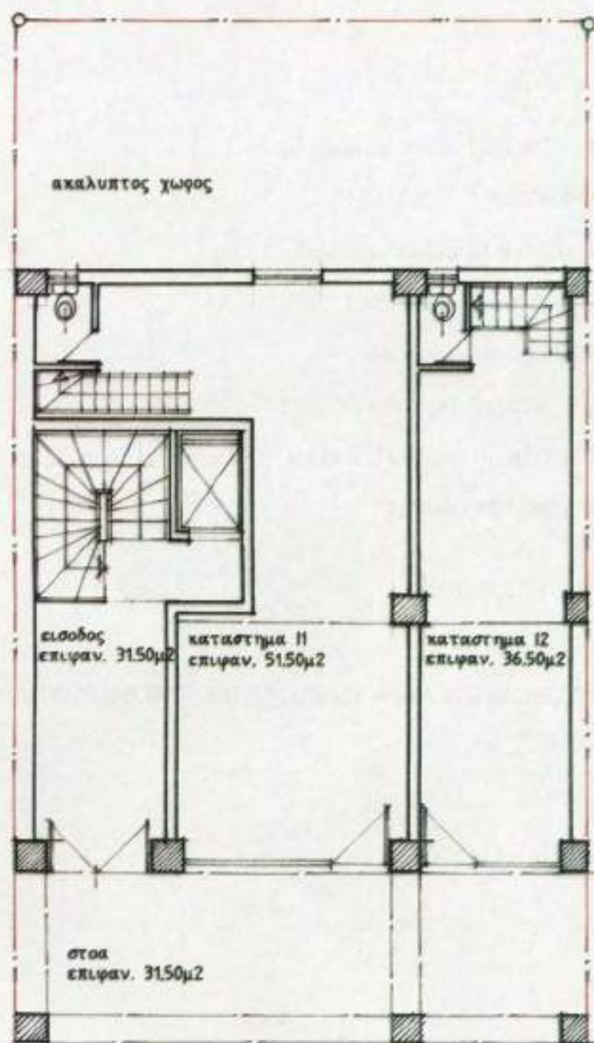
6.18.1. Κάτοψη ισογείου κλιμ.1: 60
