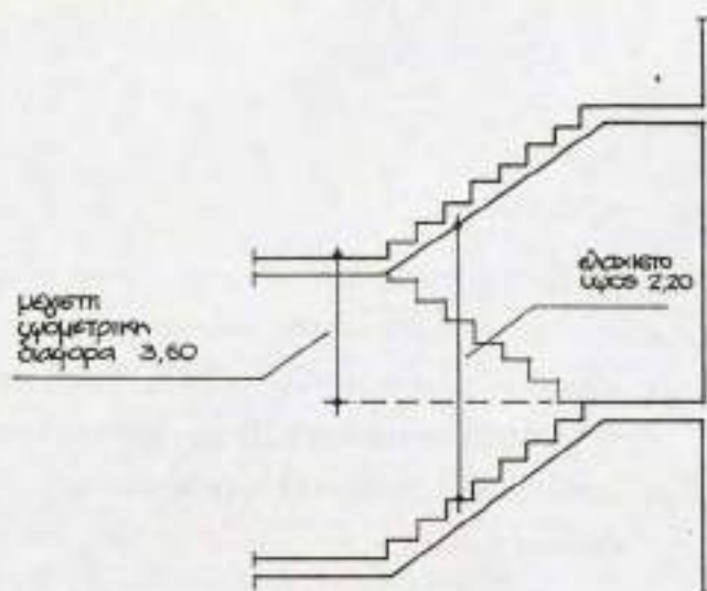
5.5. Τομή κλιμακαστασίου
