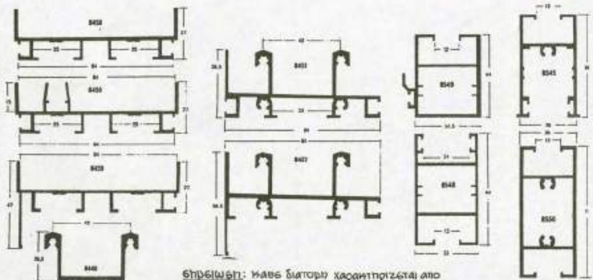
5.35. Διατομές αλουμινίου
