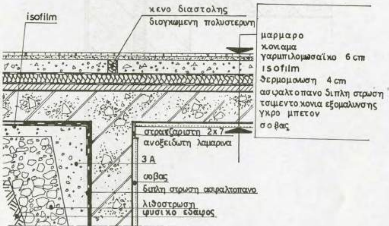
7.45. Λεπτομέρειες διάτρωσης δαπέδων εσωτερικού χώρου
