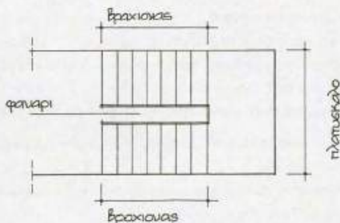
5.3.2. Κάτοψη «λιμακωστασίου»
