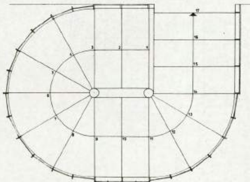
ΚΑΤΩΗ ΚΑ 1: 10
