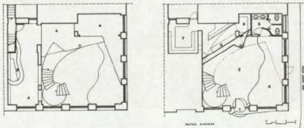
6.15.1. Κατόψεις από το εσωτερικό του καταστήματος
