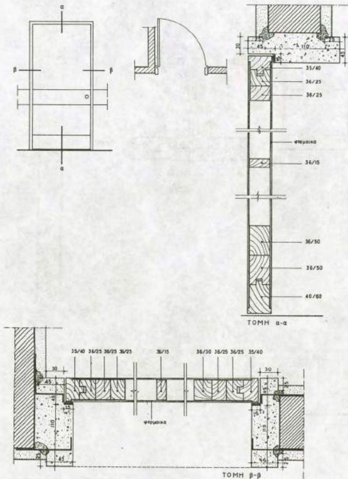
7.32. Λεπτομέρεια μονωμένης ανοιγόμενης πόρτας
