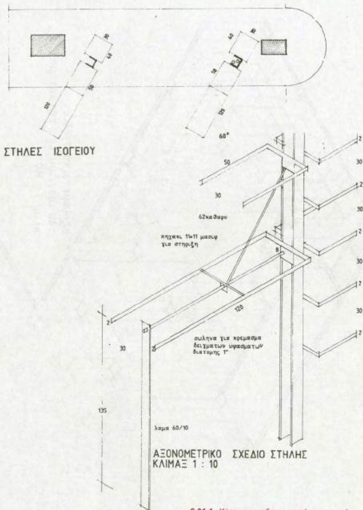
6.21.4. Κάτοψη και αξονομετρικό κρεμαστρών
