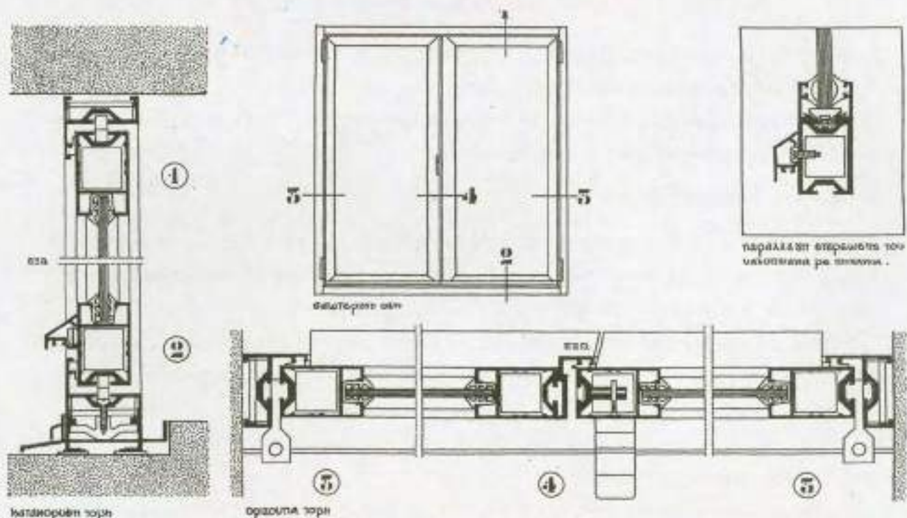
5.34.2. Διφυλλο ανοιγόμενο παράθυρο από αλουμίνιο που στρέφεται γύρω από κατακόρυφο άξονα στην άκρη του
