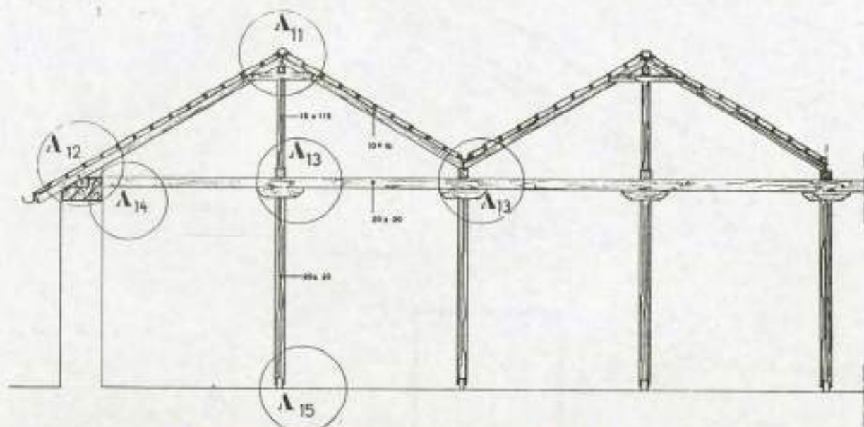
5.41. Τομή υπόστεγου που καλύπτεται από δίδυμη δýρριχτη στέγη.
