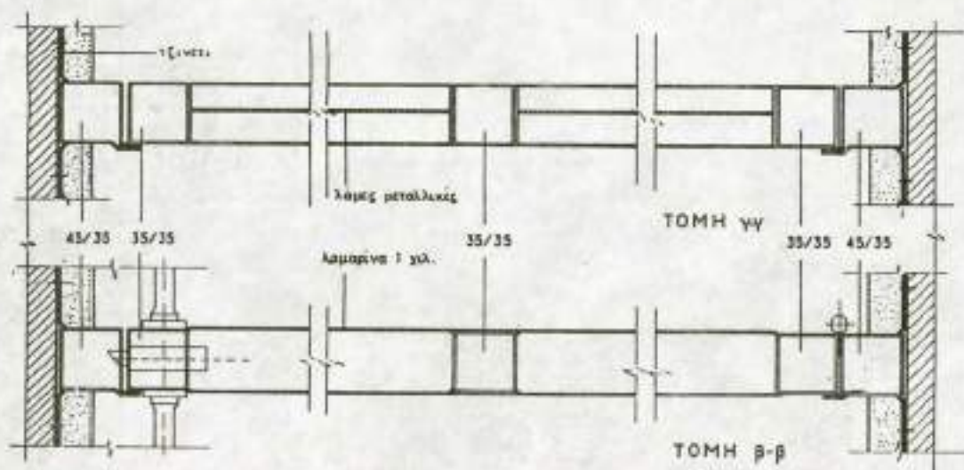
7.55. Λεπτομέρεια μονόφυλλης μεταλλικής πόρτας με περαιδες (γρίλλες) εξαερισμού
