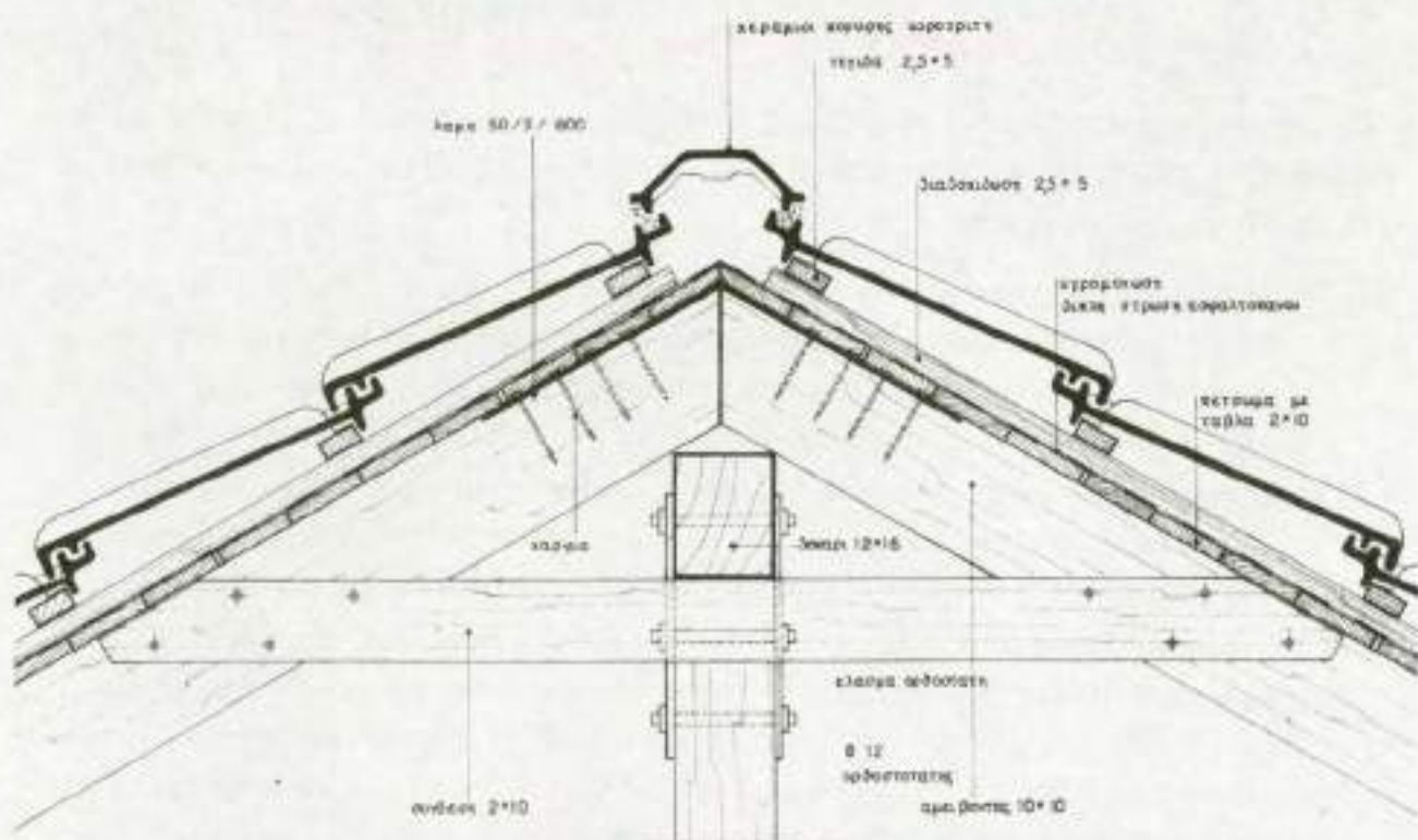
5.41.1. Λεπτομέρεια Α11: κορυφή
