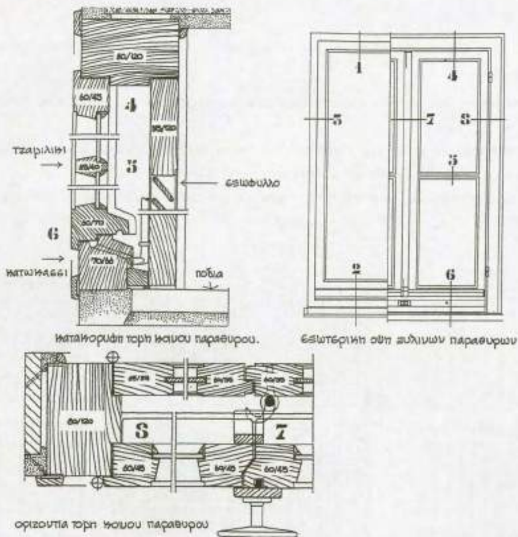
5.28. Λεπτομέρειες διφυλλου (με εξώφυλλο γαλλικού τύπου), ξύλινου παραθύρου
