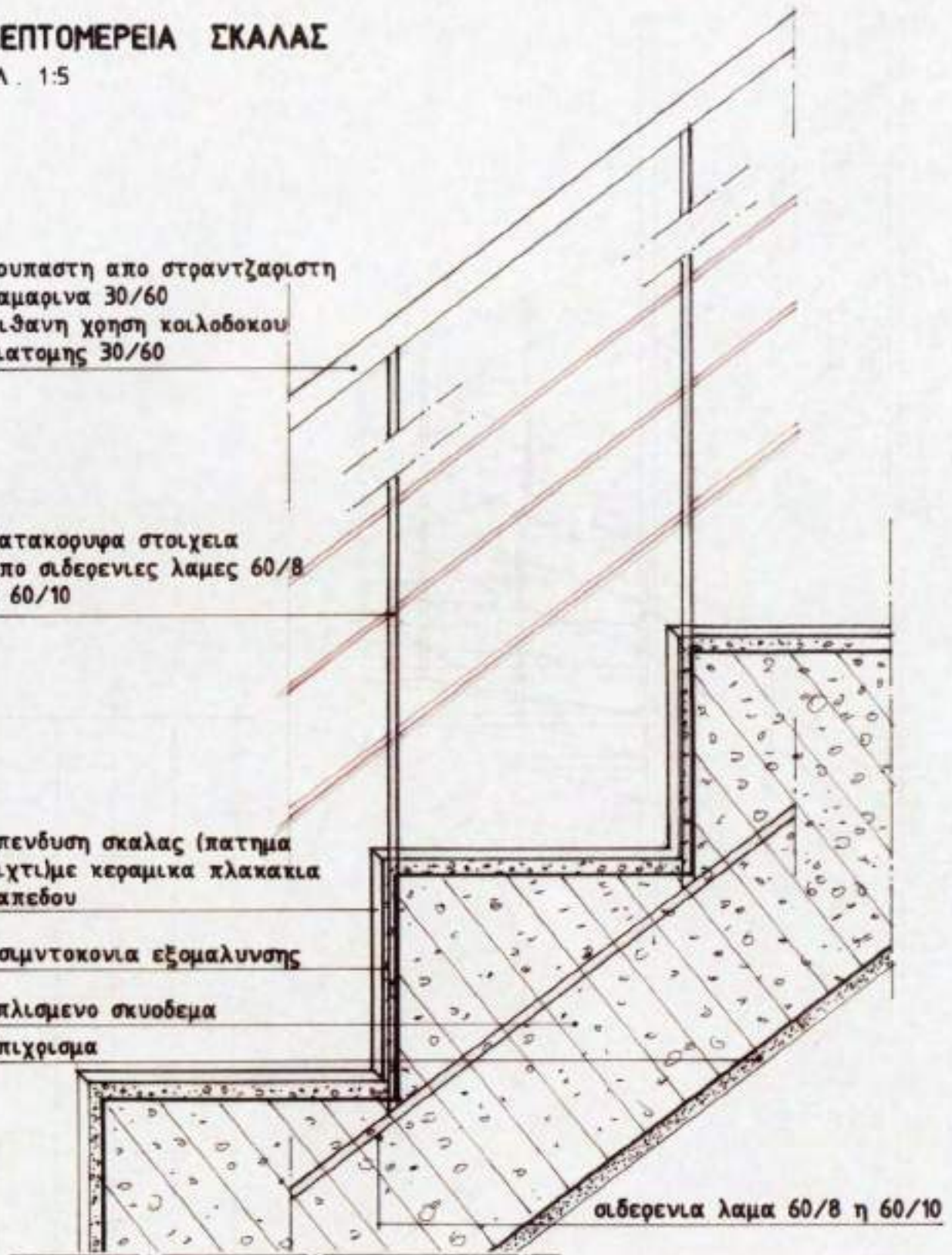
7.26. Κατασκευαστικές λεπτομέρειες σκάλας
