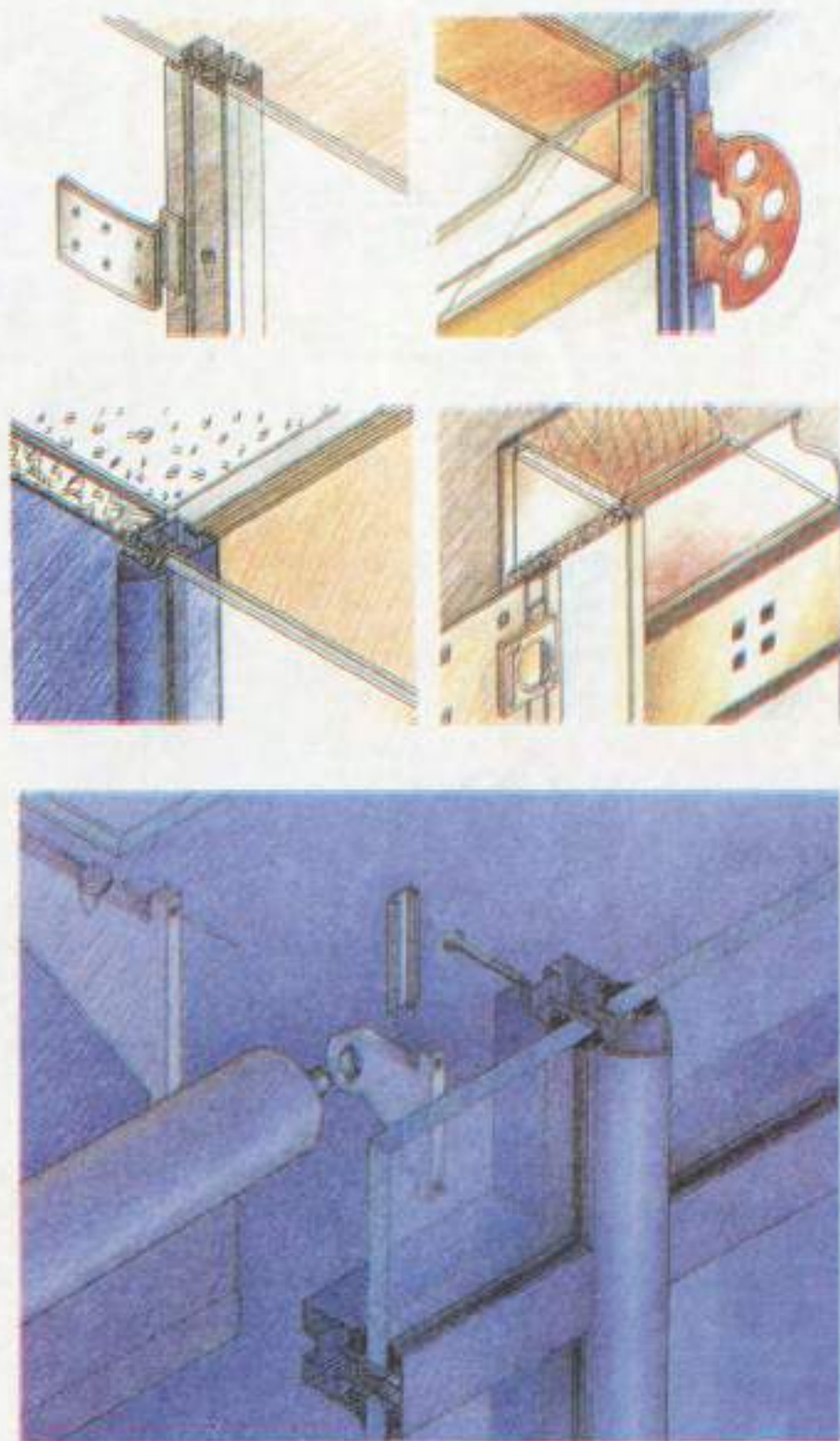
6.5. Στοιχεία εξοπλισμού
