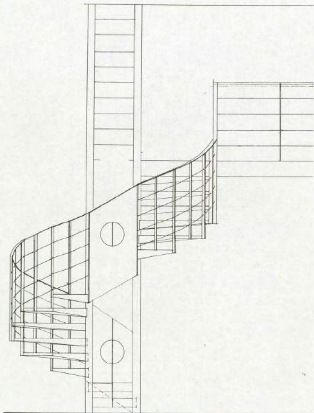
6.20.2. Όψη κλιμακοστάσιου
