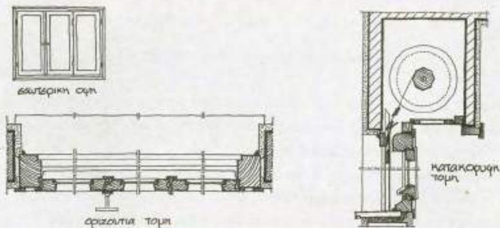
5.29. Λεπτομέρεια κατασκευής ρολού
