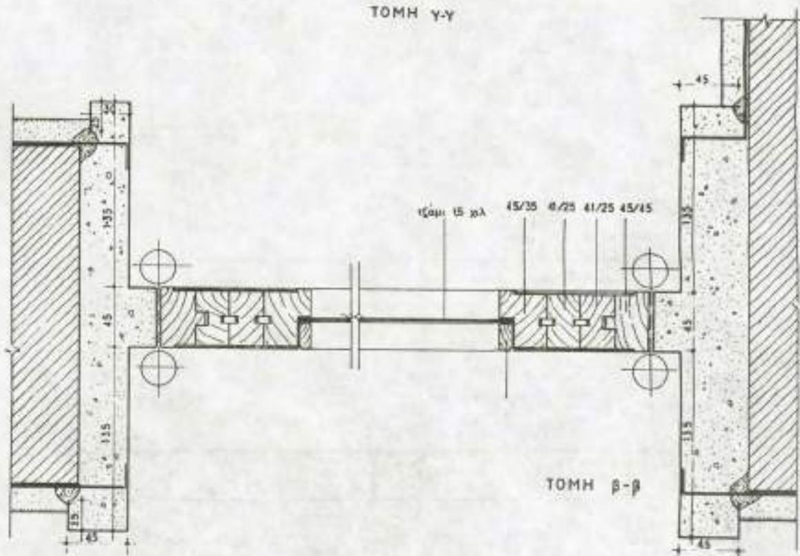
TOMH γ-γ
