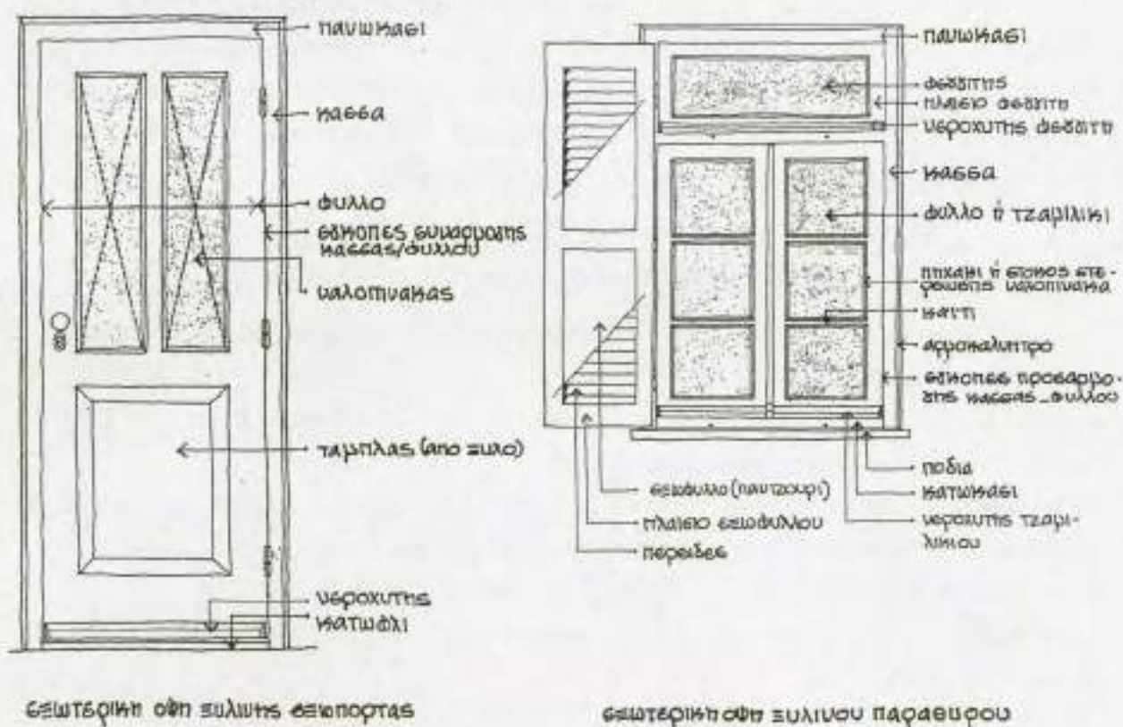
5.26. Τα κυριότερα κατασκευαστικά στοιχεία από τα οποία αποτελείται μια εξωτερική πόρτα και ένα παράθυρο
