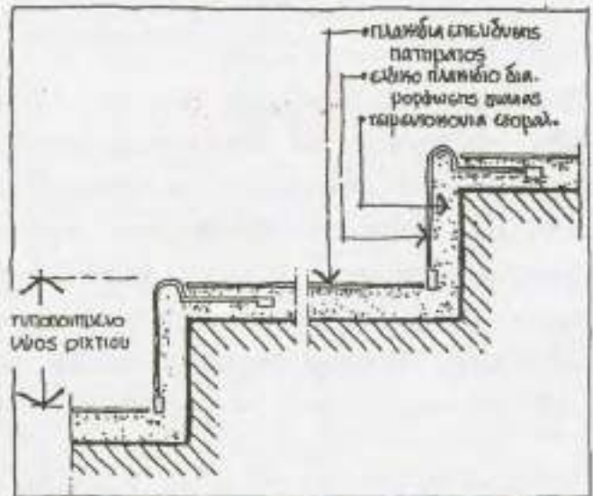
5.12.1. Επίνδυση σκάλας με κεραμικά πλακίδια
